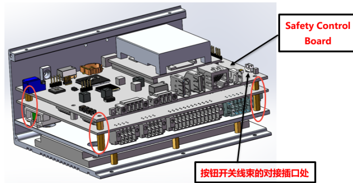
图 3-30: 拆除 Safety Board 板上的螺钉
