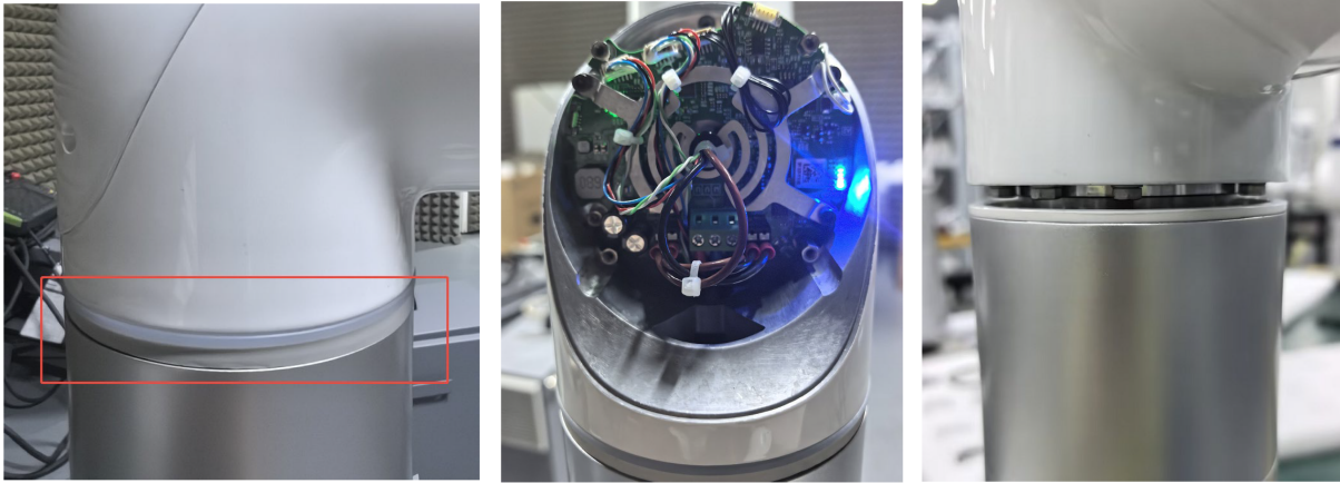
图 3-5: 取下橡胶环
