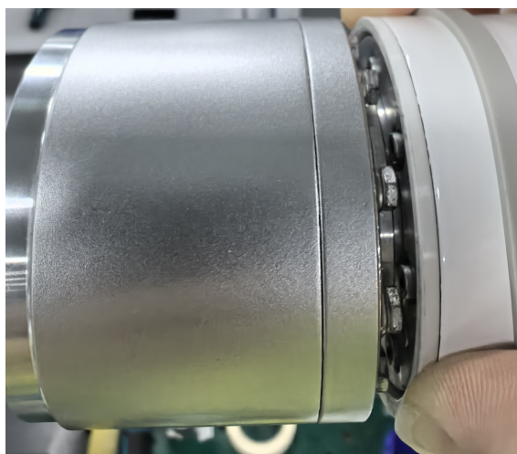
图 3-19: 取下橡胶环
