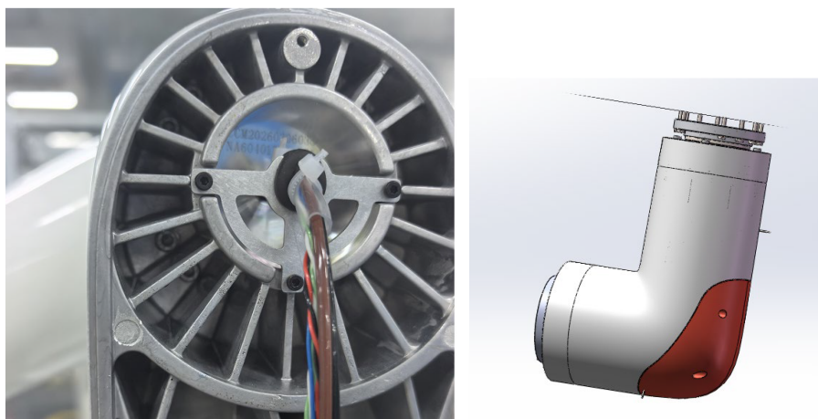
图 3-10: M3 螺钉
