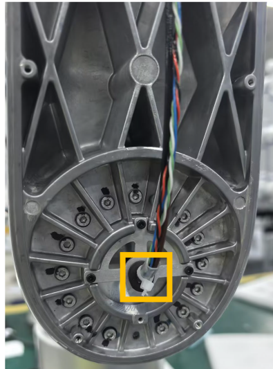
图 3-25: 连杆线缆安装
