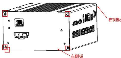
图 3-28: 拆除左右侧板
