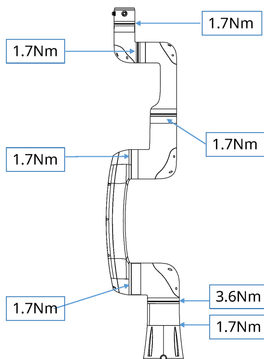
图 3-1: 各关节扭矩图
