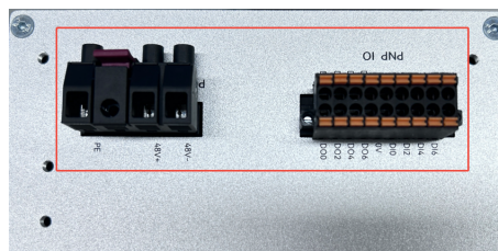
图 3-27: 拆除 I/O 接口插头 (2)
