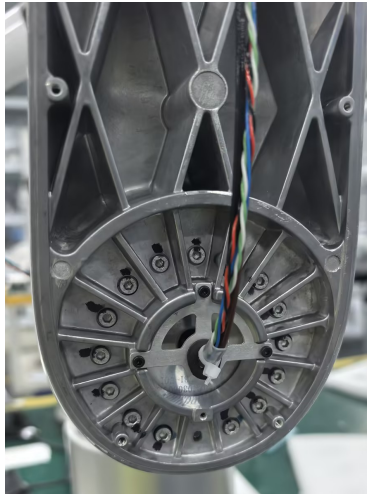
图 3-8: M3 螺钉
