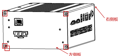
图 3-36: 拆除左右侧板
