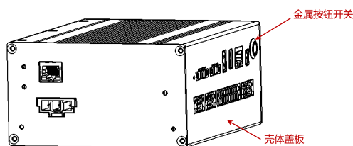
图 3-29: 拆除壳体盖板
