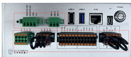
图 3-26: 拆除 I/O 接口插头 (1)
