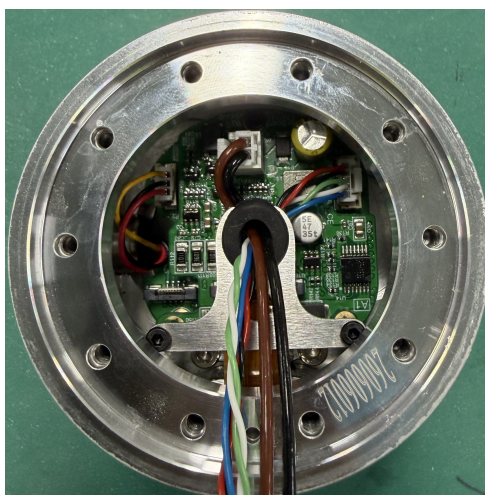
图 3-20: 连接末端法兰和手腕关节的电线
