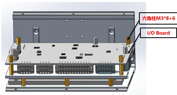
图 3-32: 拆除六角柱
