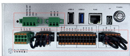
图 3-34: 拆除 I/O 接口插头 (1)
