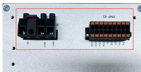
图 3-35: 拆除 I/O 接口插头 (2)
