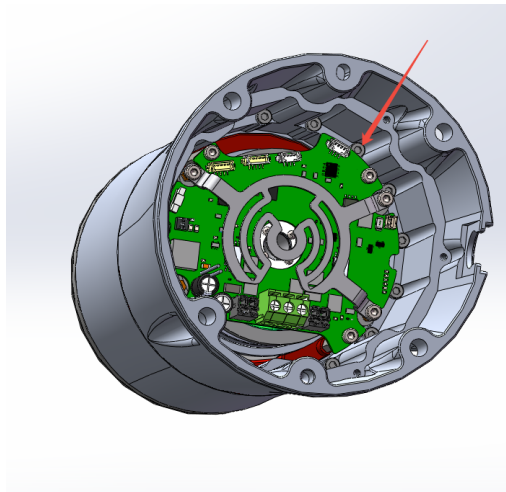
图 3-3: 断开基座与基座关节
