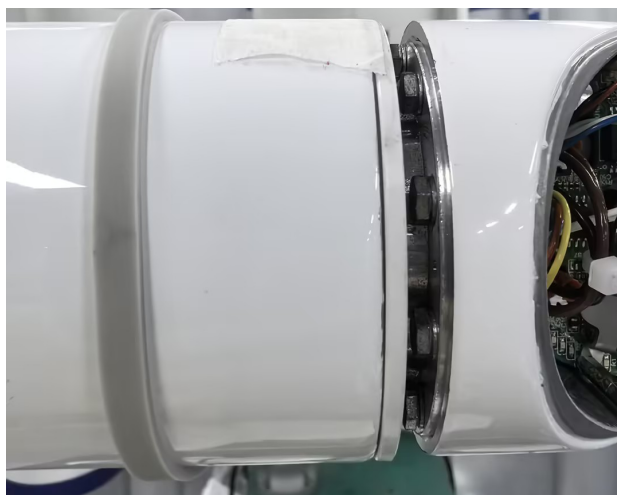
图 3-16: 取下橡胶环
