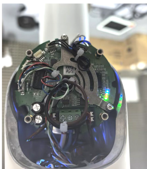
图 3-24: 接线和扎线
