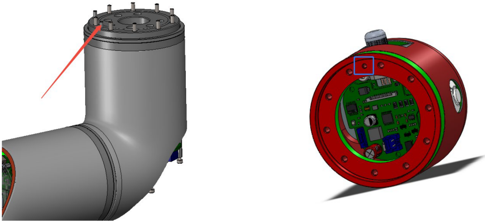
图 3-21: 连接末端法兰和手腕关节
