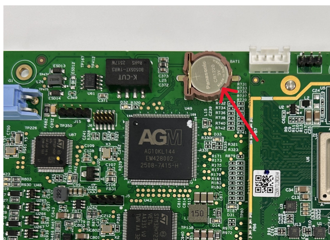
图 3-39: 纽扣电池安装方向
