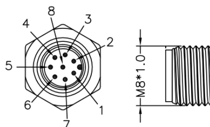
图 2-41: 机器人末端 I/O 航空插头接口
