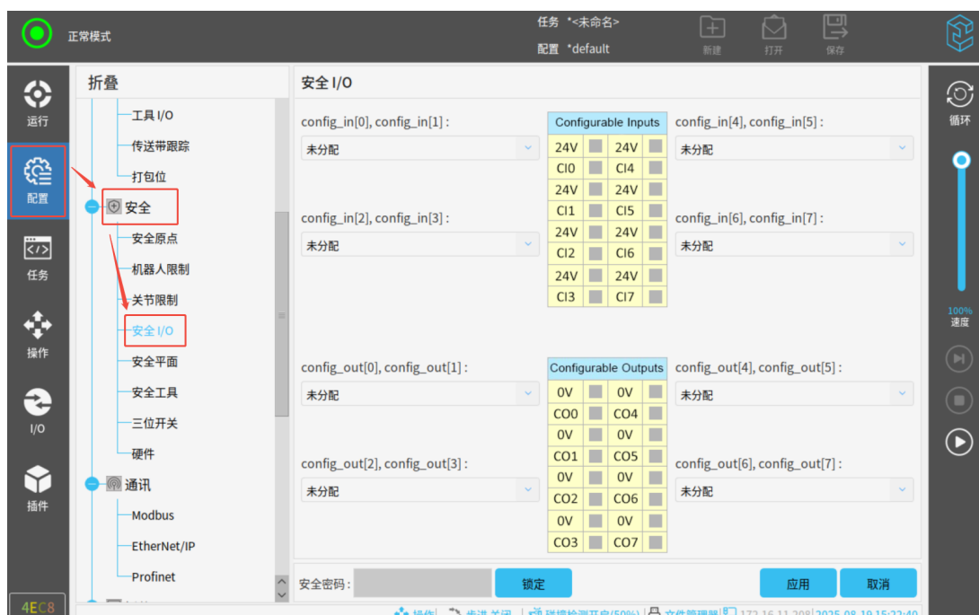
图 3-79: 安全 I/O
