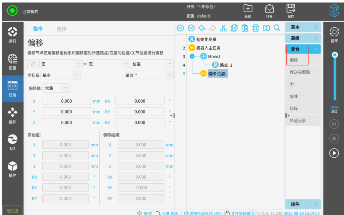
图 3-135: 偏移
