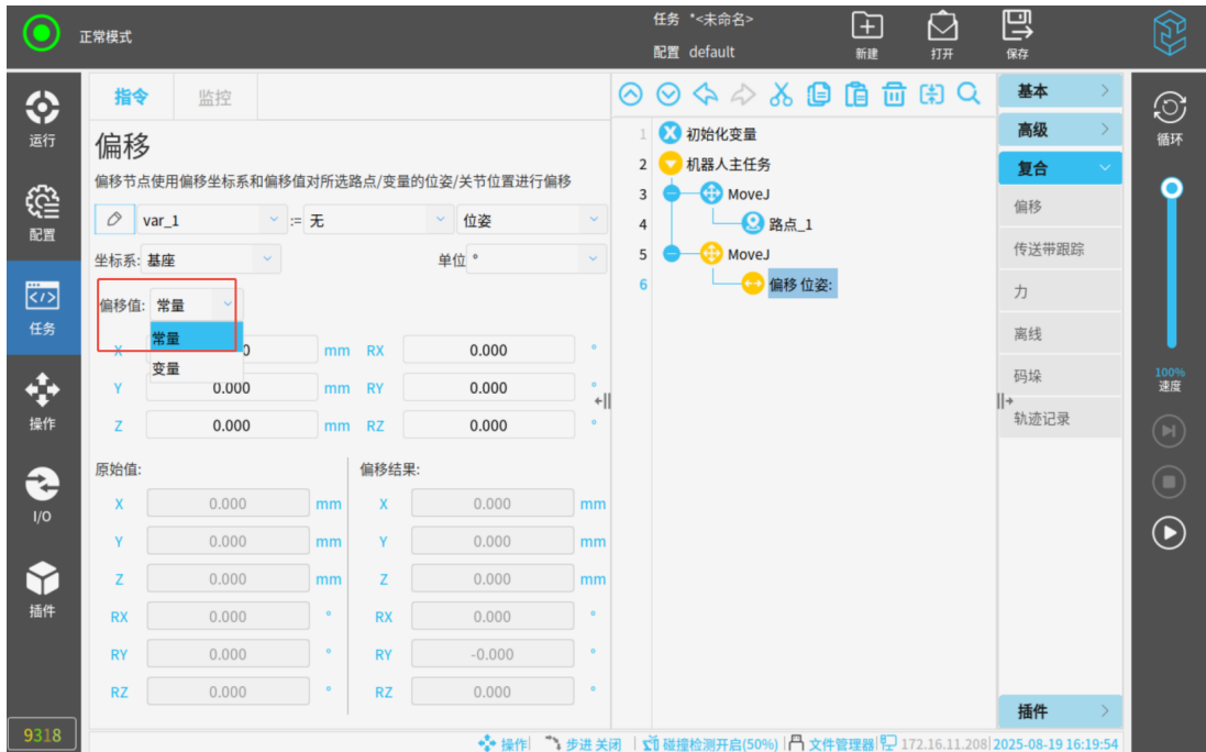
图 3-145: 指定偏移值
