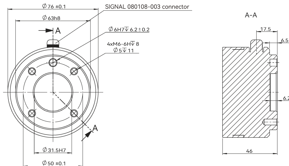
图 2-5: ES66 机器人工具法兰安装尺寸 (单位: mm)
