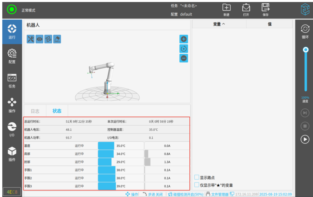
图 3-39: 状态
