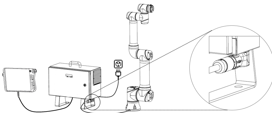
图 1-7: 整机安装-本体电缆锁定
