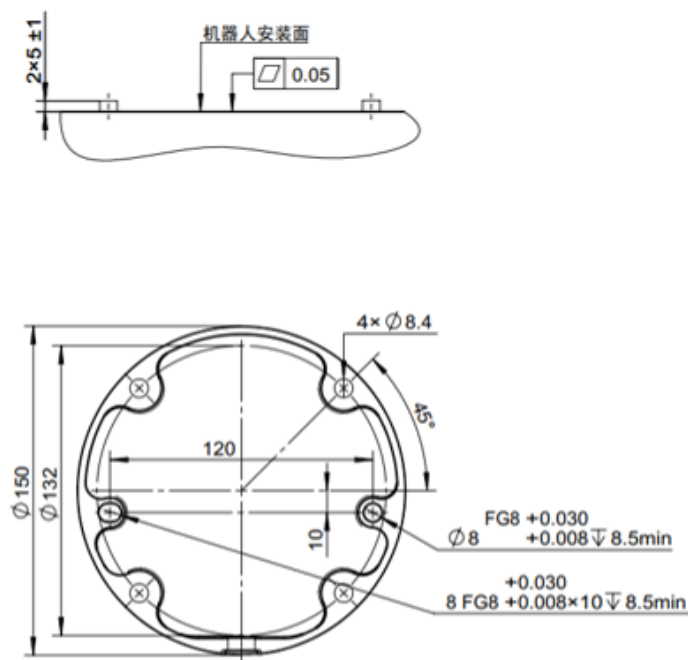
图 2-4: ES66 机器人基座安装尺寸（单位：mm）
