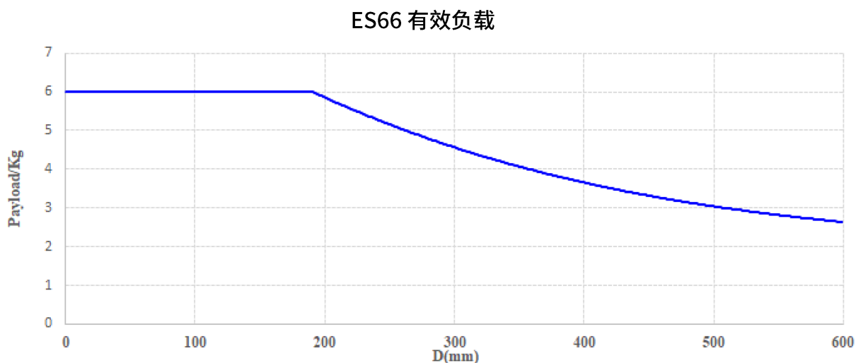
图 2-6: ES66 机器人有效负载
