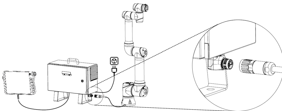
图 1-5: 整机安装-本体电缆未连接
