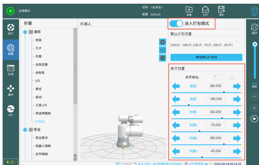
图 3-74: 打包模式
