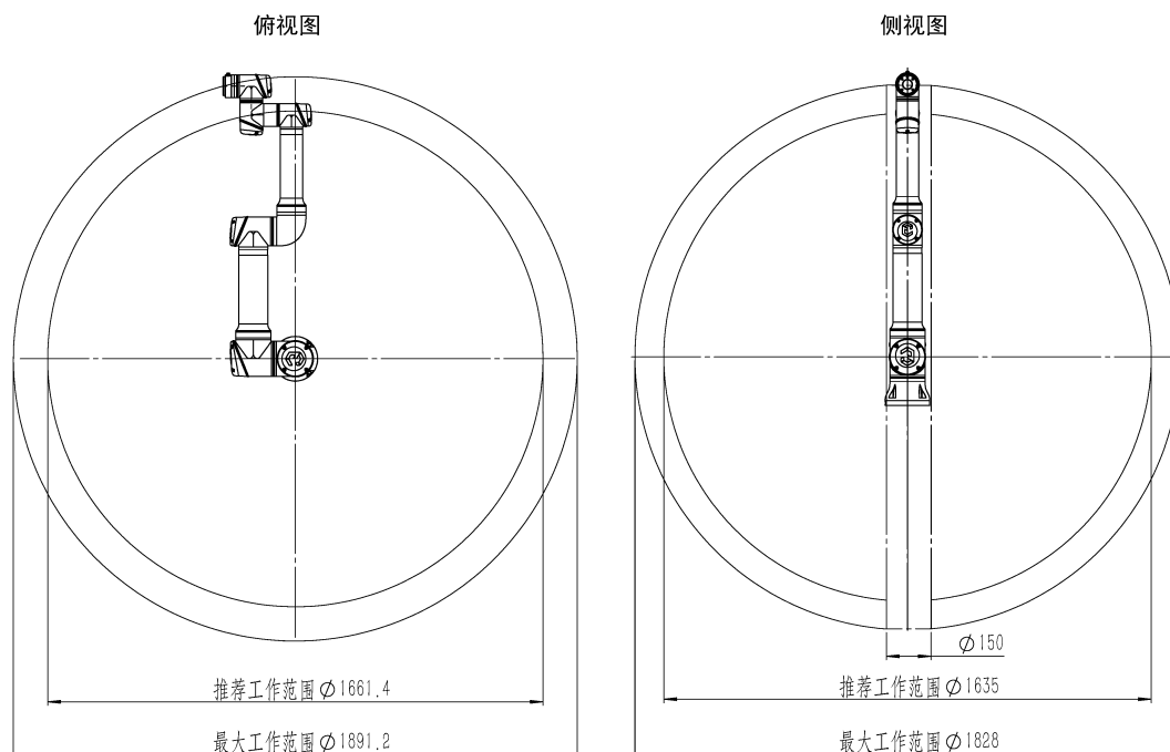
图 2-2: ES66 机器人工作空间（单位：mm）
