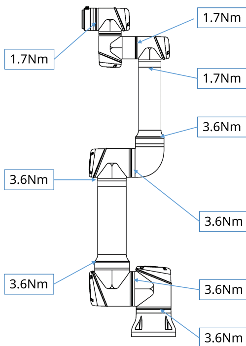
图 3-7: 各关节扭矩图
