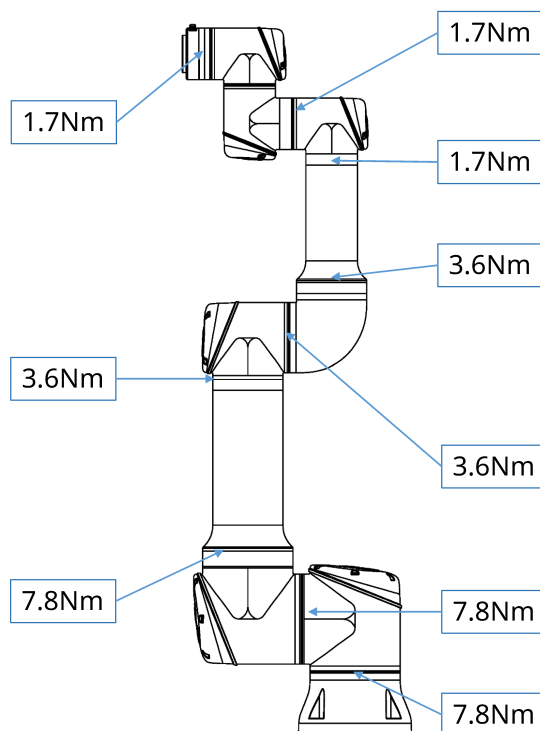
图 3-7: 各关节扭矩图
