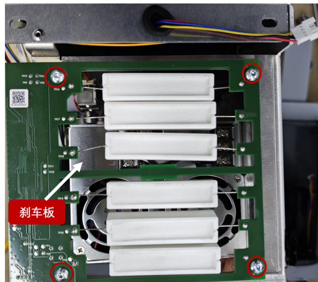
图 3-31: 取下刹车板
