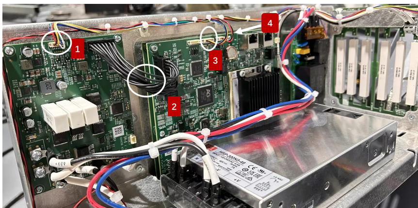
图 3-27: 电源板、刹车板到 Safety I/O 板的线缆位置
