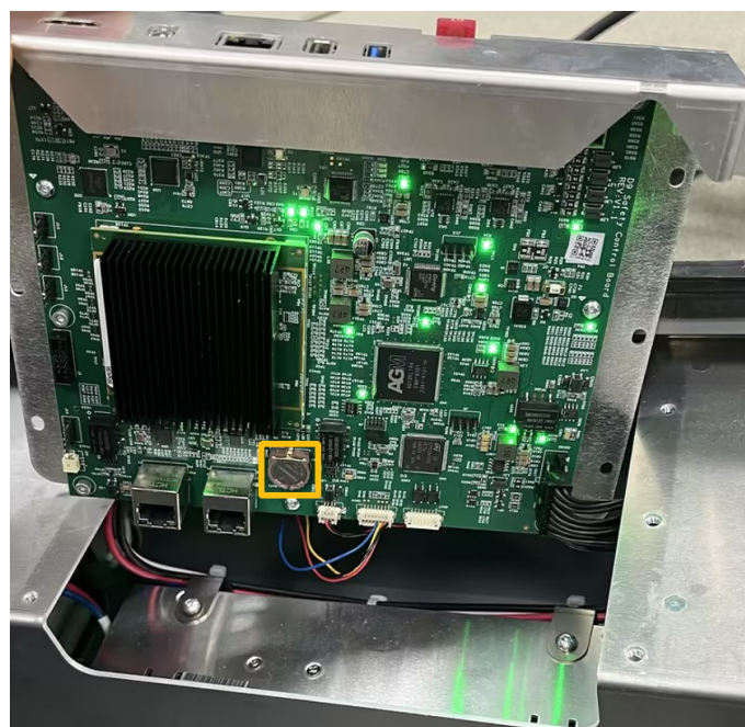
图 3-34: 纽扣电池安装位置
