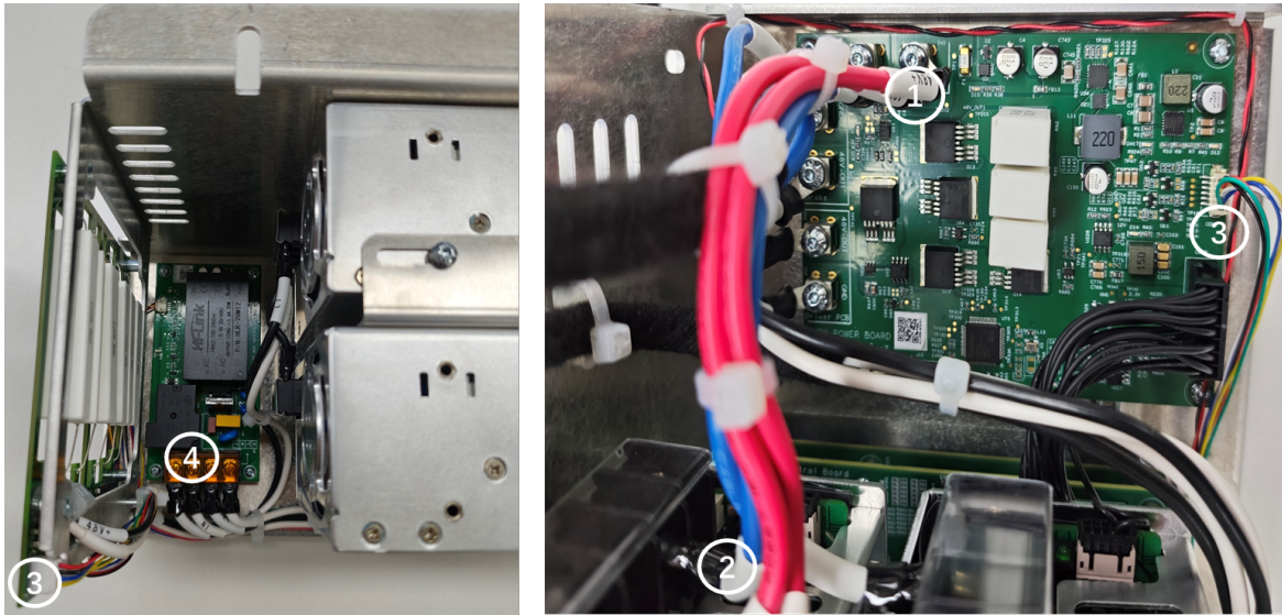
图 3-26: 控制柜上的电源连接线位置
