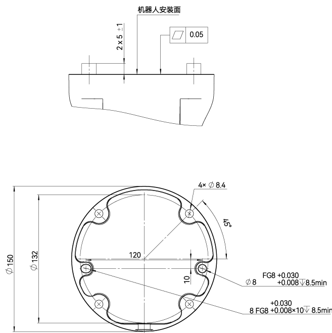
图 2-4: CS68 机器人基座安装尺寸（单位：mm）
