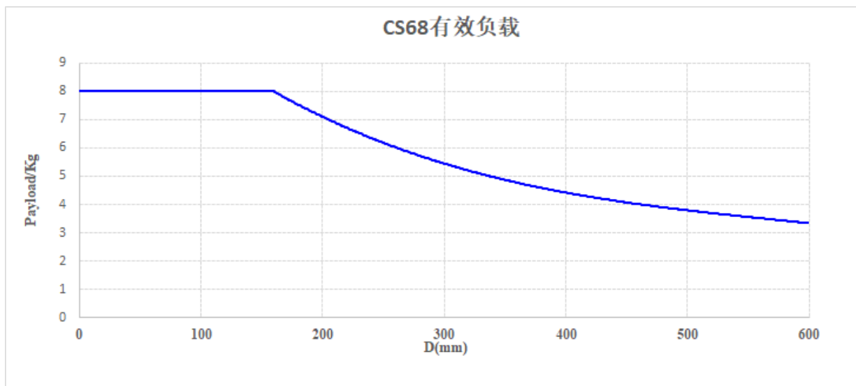
图 2-7: CS68 机器人有效负载
