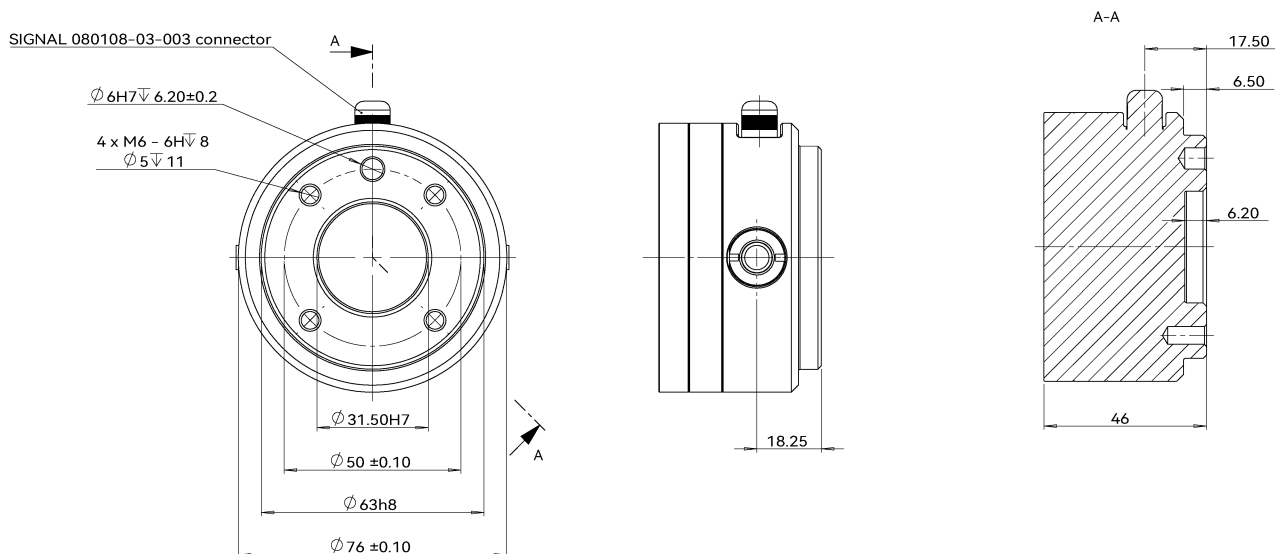
图 2-5: CS68 机器人工具法兰安装尺寸 (单位: mm)
