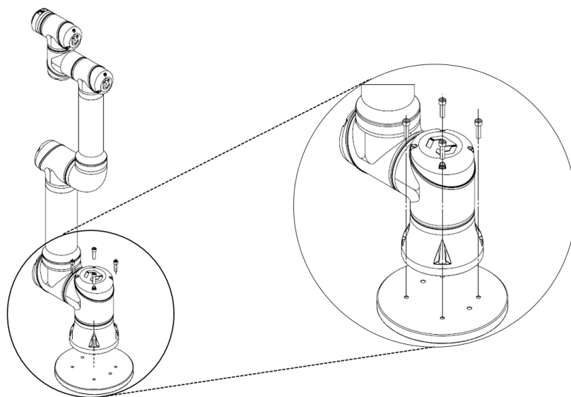
图 1-3: 本体安装
