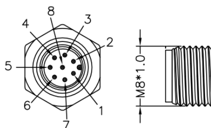
图 2-42: 机器人末端 I/O 航空插接口
