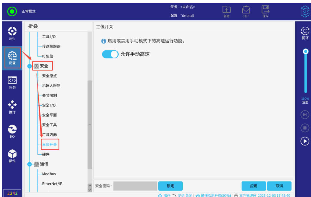
图 3-97: 三位开关
