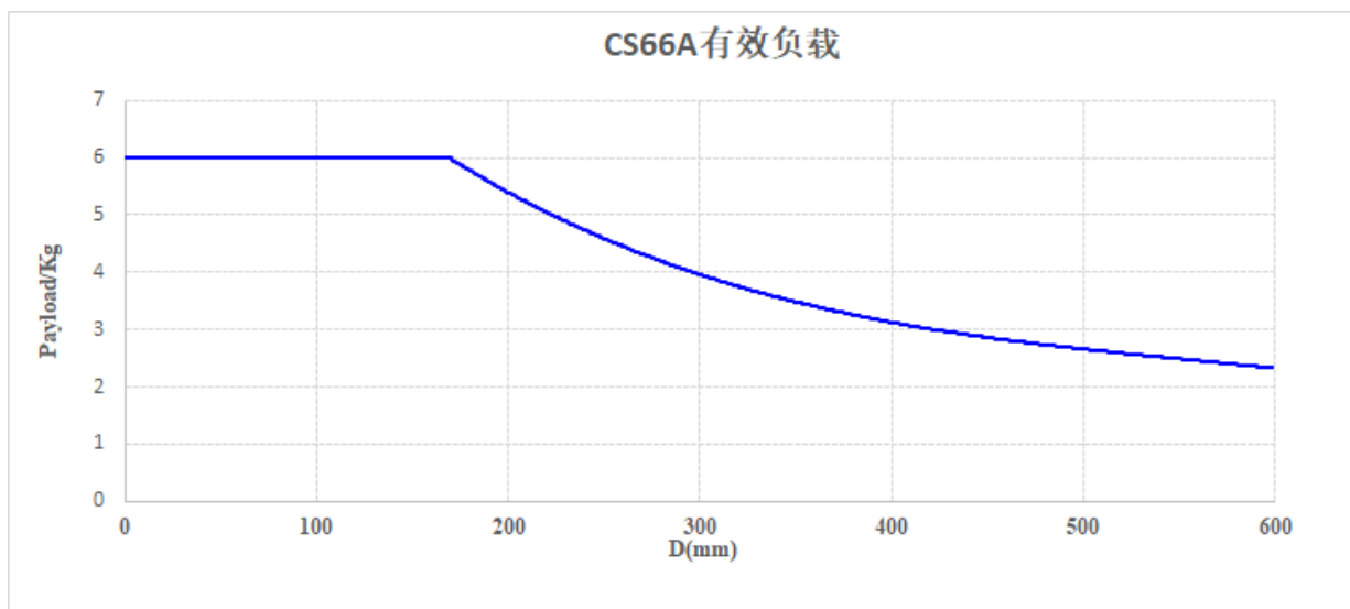
图 2-7: CS66A 机器人有效负载
