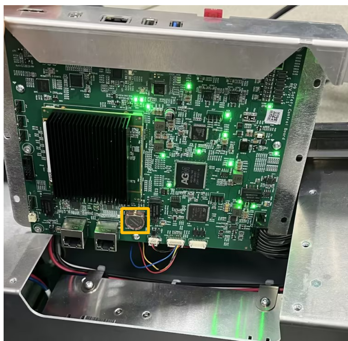
图 2-9: 纽扣电池安装位置
