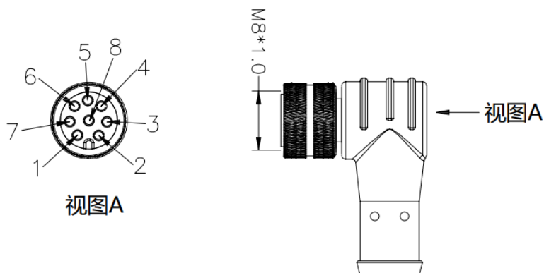
图 2-43: 用户航插焊线
