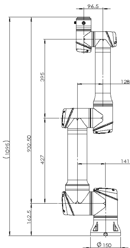
图 2-1: CS66A 机器人机械尺寸（单位：mm）
