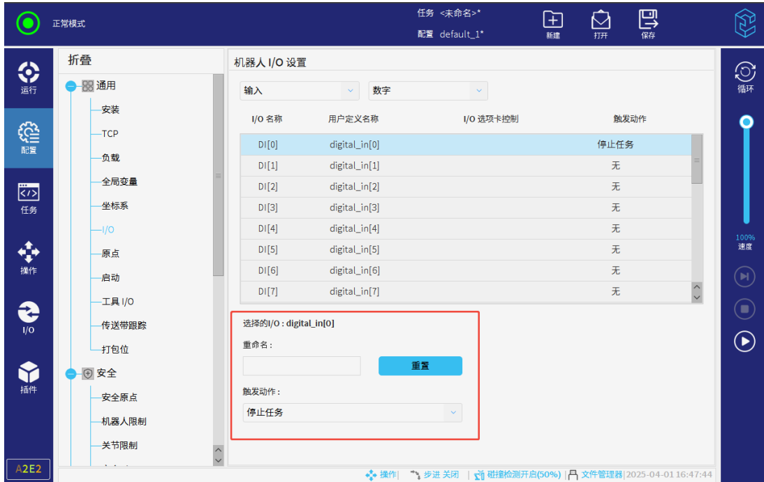
图 3-65: 数字输入信号
