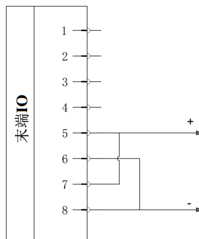
图 2-46: 双针模式 2 接线
