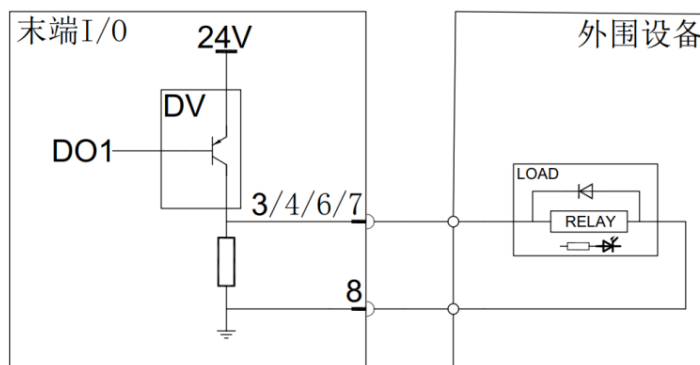
图 2-49: PNP 模式
