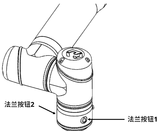
图 2-6: CS66A 机器人末端法兰按钮
