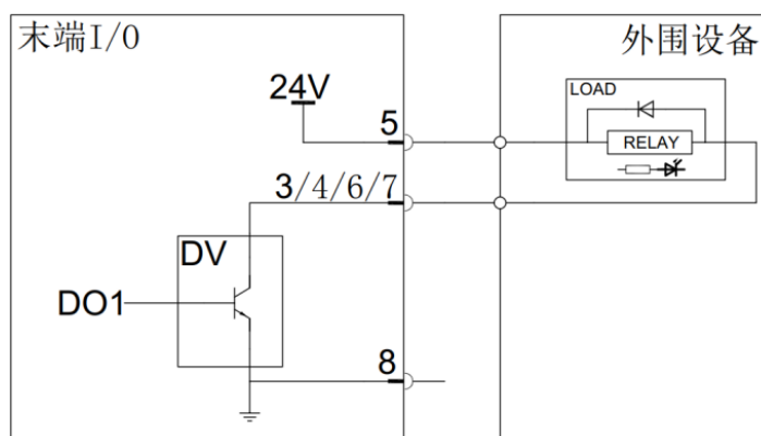
图 2-48: NPN 模式
