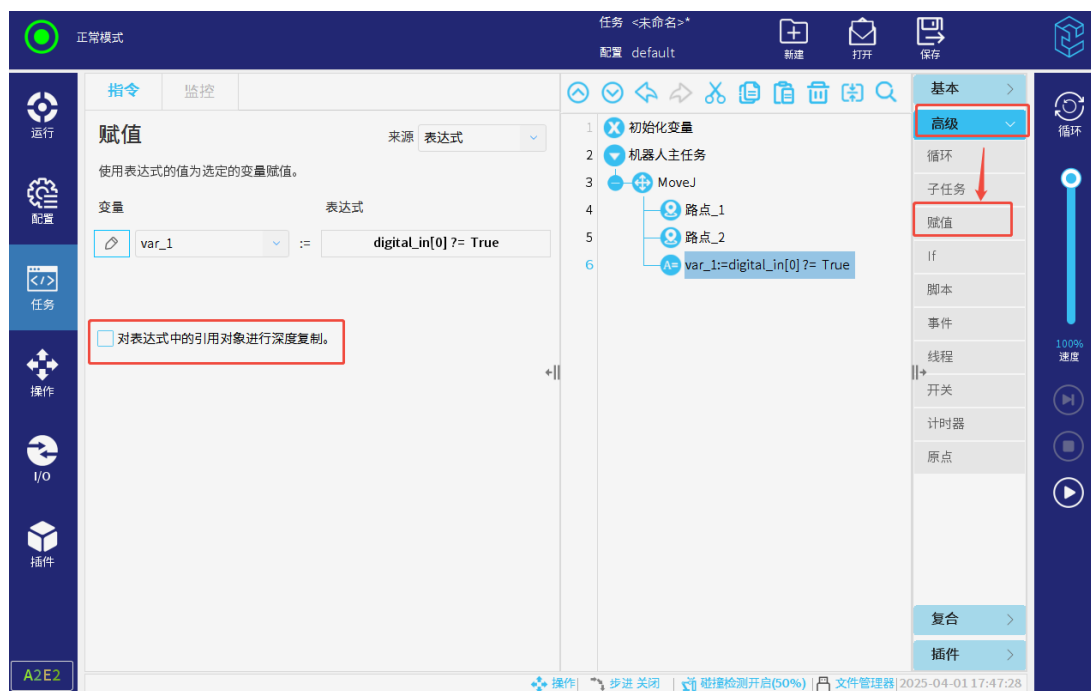
图 3-129: 赋值
