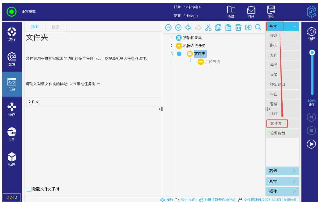
图 3-125: 文件夹
