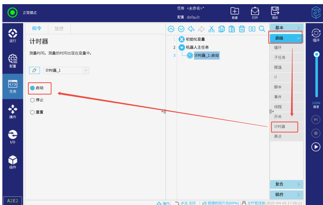
图 3-135: 计时器
