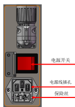
图 2-10: 电源输入插座
