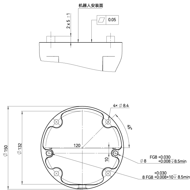
图 2-4: CS66A 机器人基座安装尺寸 (单位: mm)
