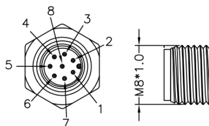
图 2-42: 机器人末端 I/O 航插接口
