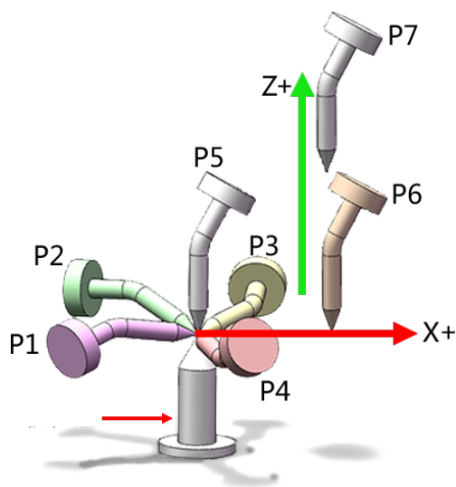
图 3-50: 三点法示教坐标系方向
