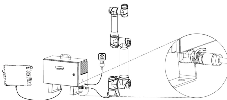
图 1-6: 整机安装-本体电缆连接
