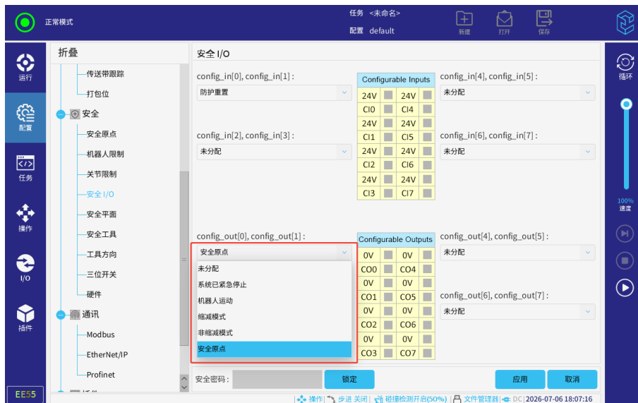
图 3-85: 为安全原点选择输出信号
