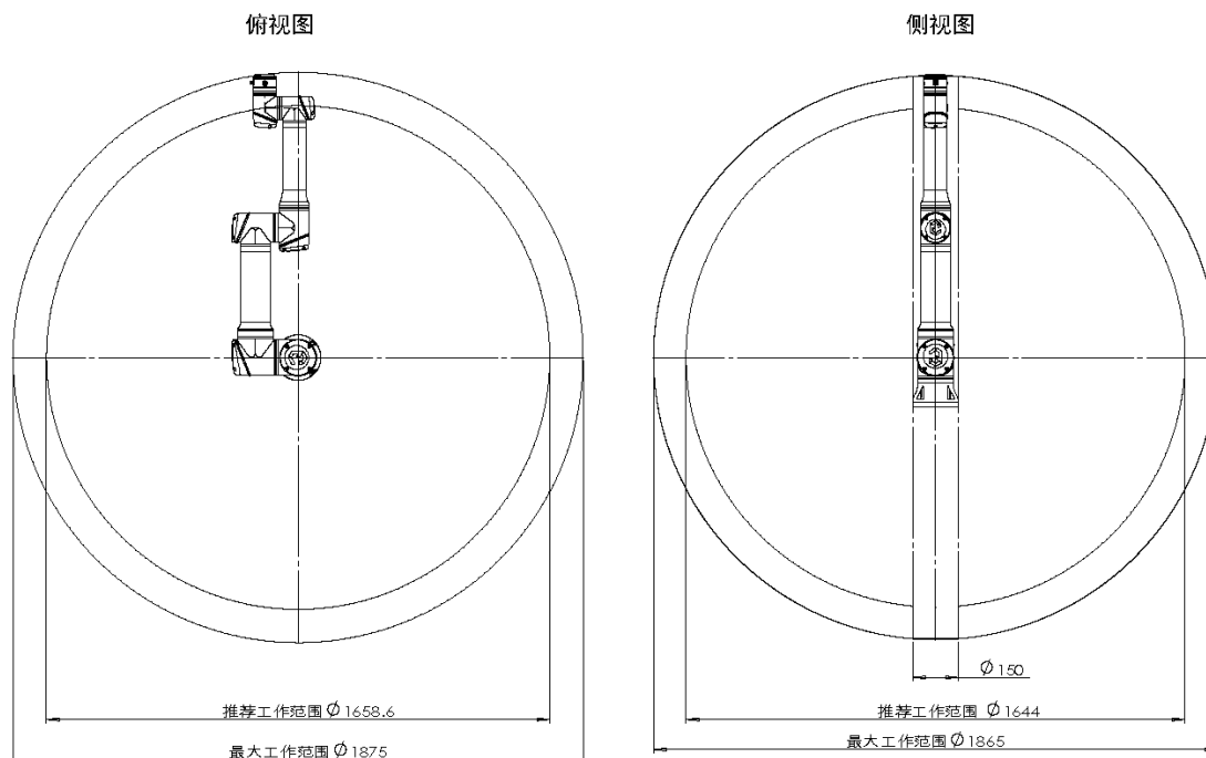
图 2-2: CS66A 机器人工作空间（单位：mm）
