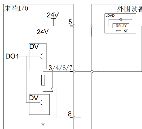
图 2-51: NPN 模式接线
