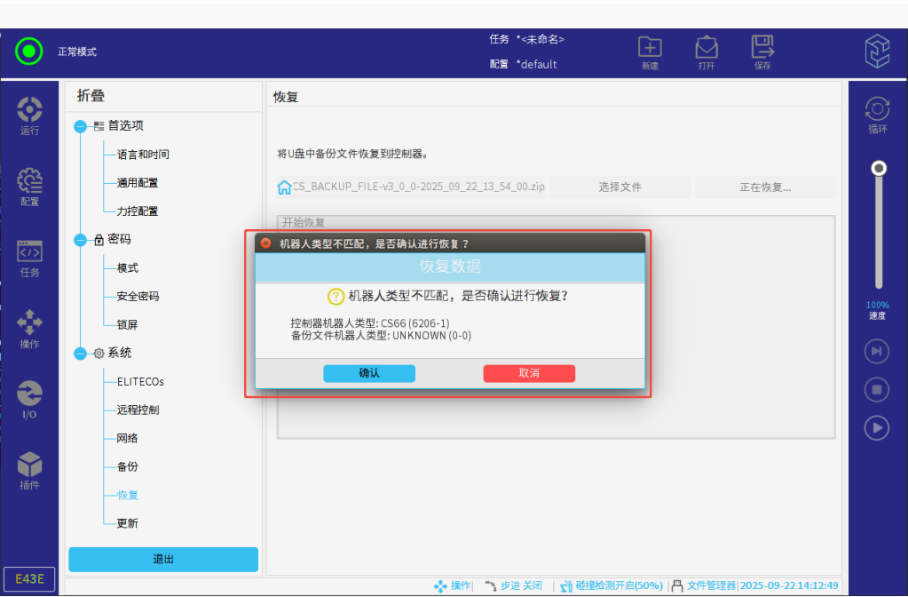
图 3-32: 机器人类型不匹配提示
