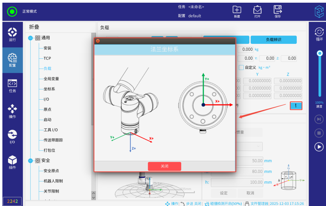
图 3-51: 法兰坐标系方向
