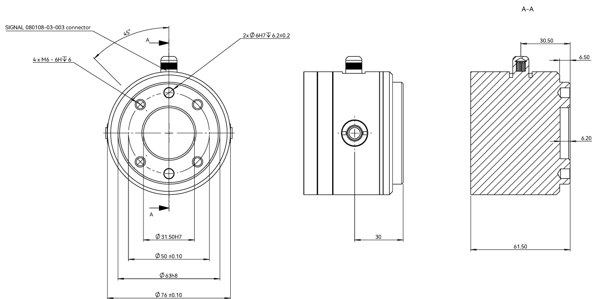
图 2-5: CS66A 机器人工具法兰安装尺寸 (单位: mm)
