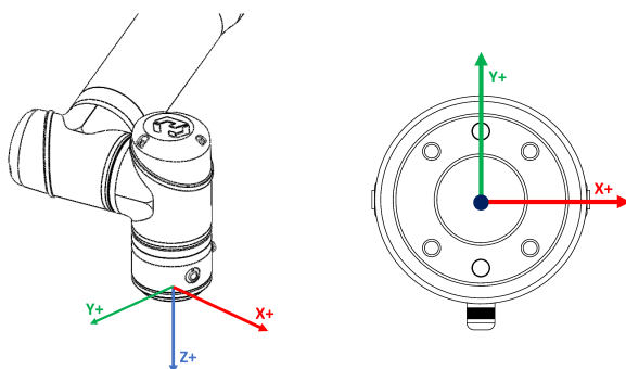
图 3-44: 工具坐标默认方向
