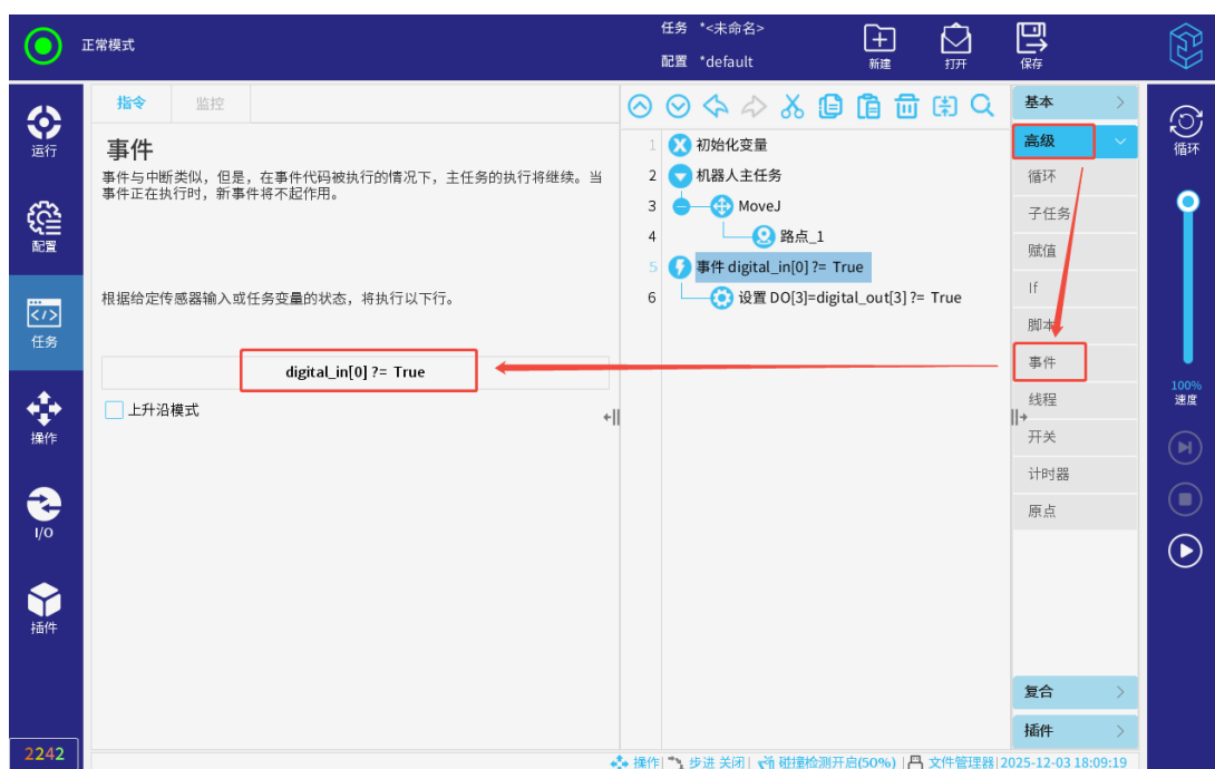
图 3-132: 事件
