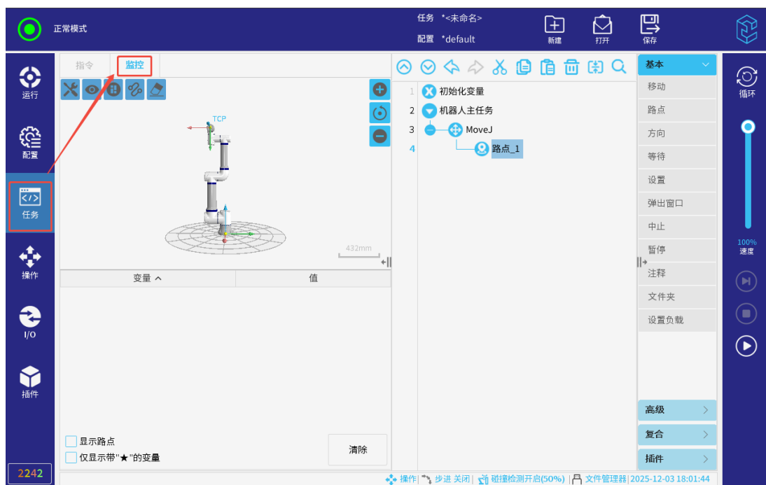
图 3-112: 监控界面
