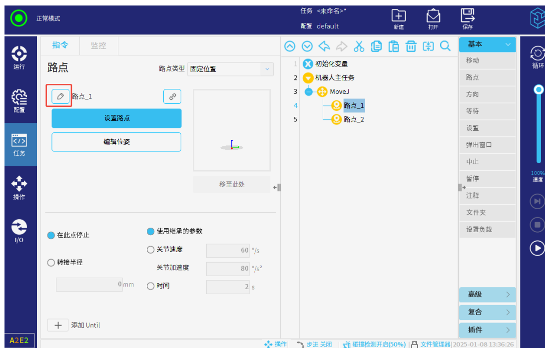
图 3-116: 重命名
