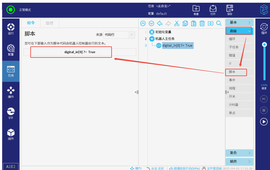
图 3-131: 脚本
