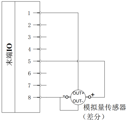
图 2-54: 模拟输入（差分）连接
