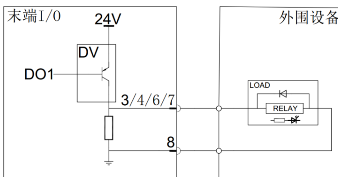
图 2-49: PNP 模式
