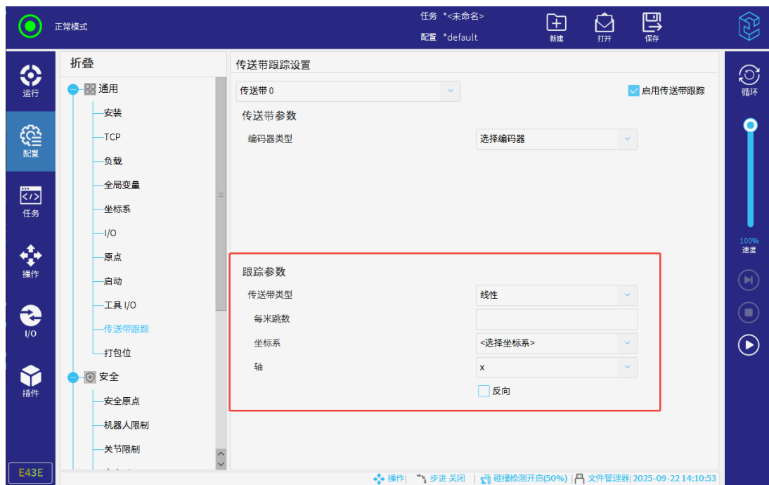
图 3-74: 设置跟踪参数
