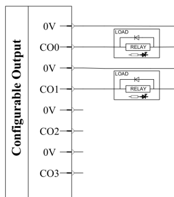
图 2-25: 配置输出接线方式
