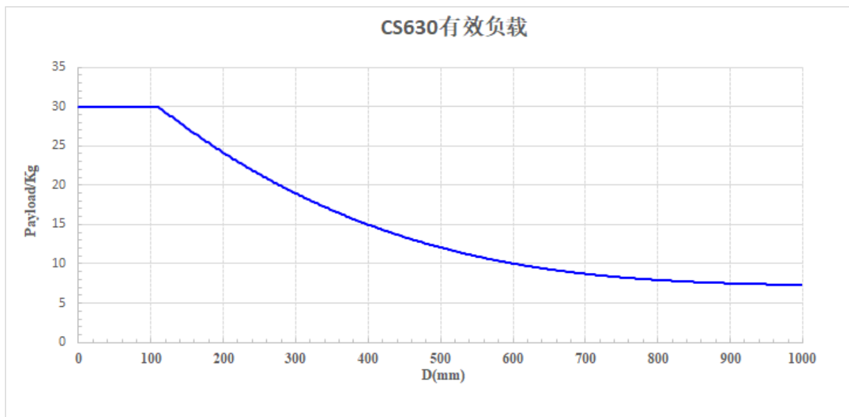
图 2-7: CS630 机器人有效负载
