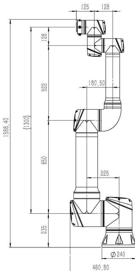
图 2-1: CS630 机器人机械尺寸（单位：mm）
