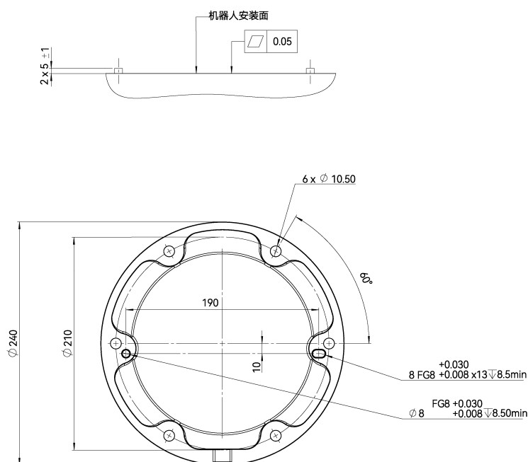
图 2-4: CS630 机器人基座安装尺寸 (单位: mm)
