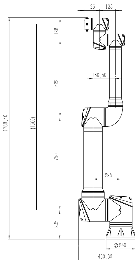
图 2-1: CS625 机器人机械尺寸 (单位: mm)
