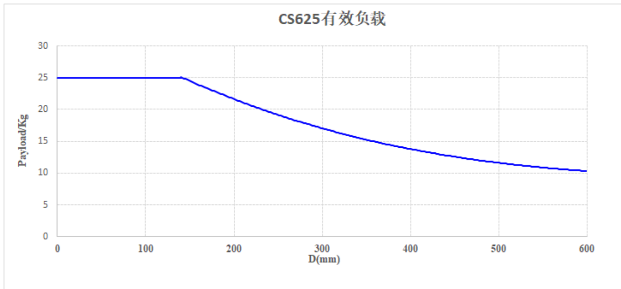
图 2-7: CS625 机器人有效负载
