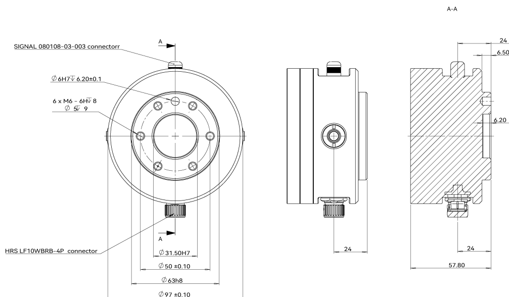
图 2-5: CS620 机器人工具法兰安装尺寸 (单位: mm)
