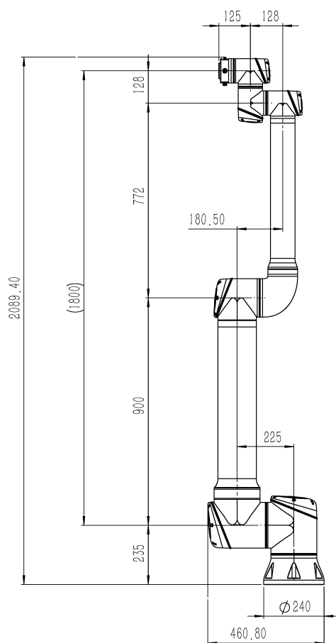
图 2-1: CS620 机器人机械尺寸（单位：mm）
