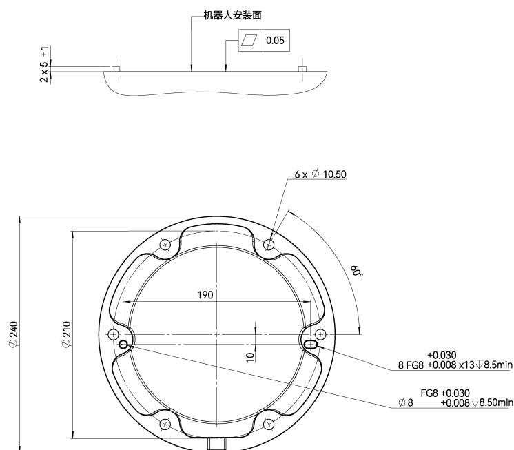
图 2-4: CS620 机器人基座安装尺寸 (单位: mm)
