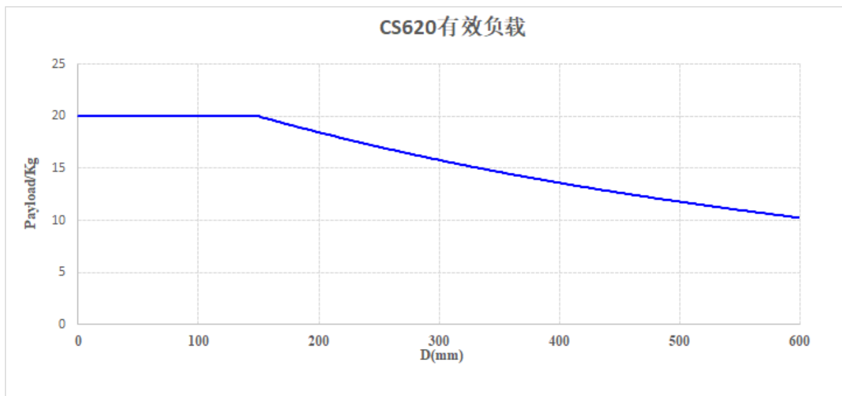
图 2-7: CS620 机器人有效负载
