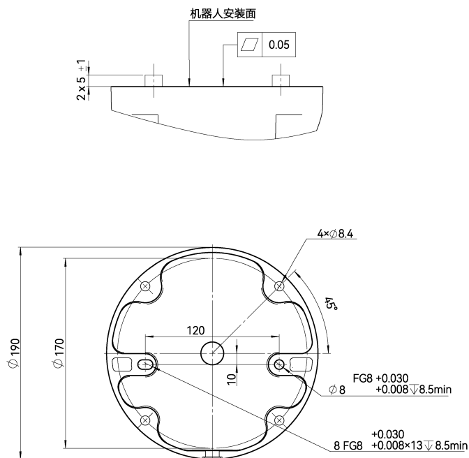
图 2-4: CS618 机器人基座安装尺寸 (单位: mm)
