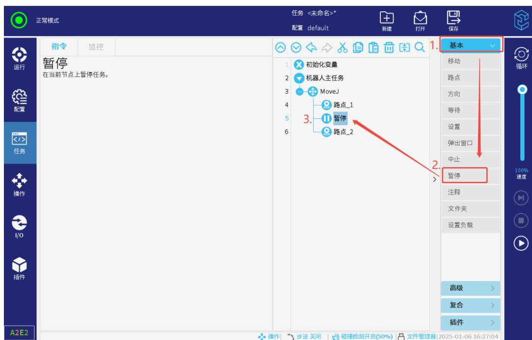
图 3-123: 暂停
