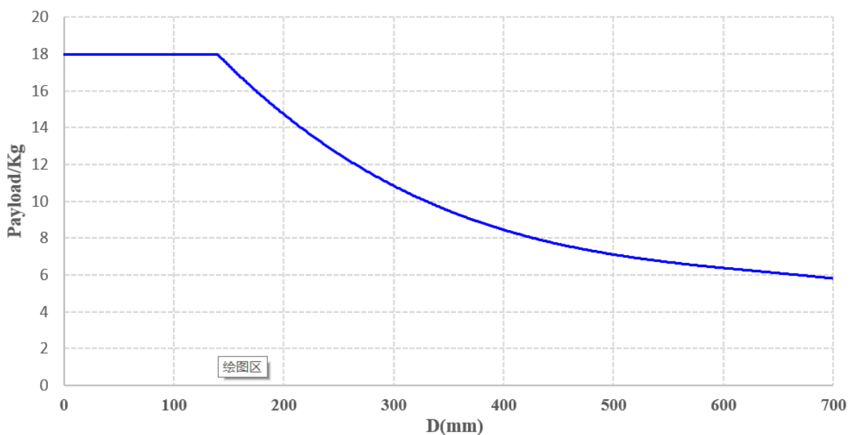
图 2-7: CS618 机器人有效负载
