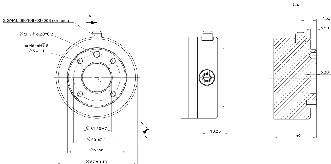
图 2-5: CS618 机器人工具法兰安装尺寸 (单位: mm)
