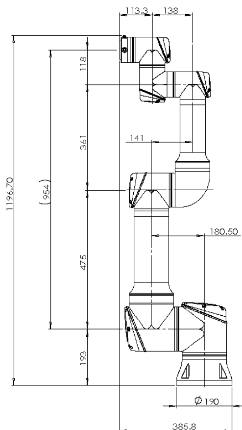
图 2-1: CS618 机器人机械尺寸（单位：mm）
