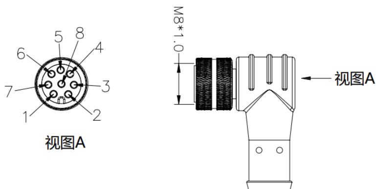
图 2-43: 用户航空插焊线
