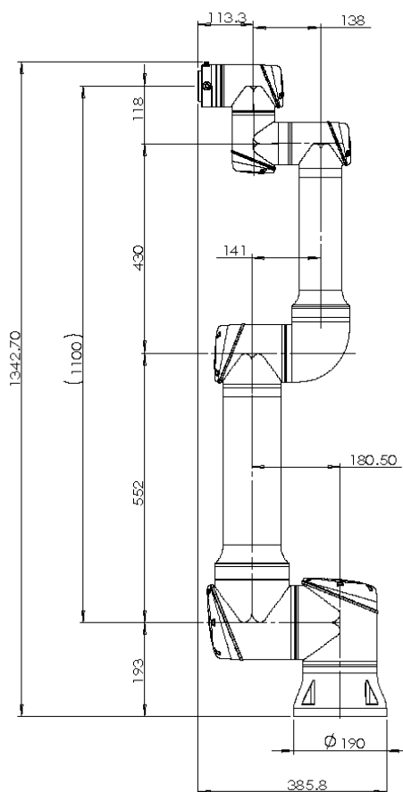
图 2-1: CS616 机器人机械尺寸 (单位: mm)
