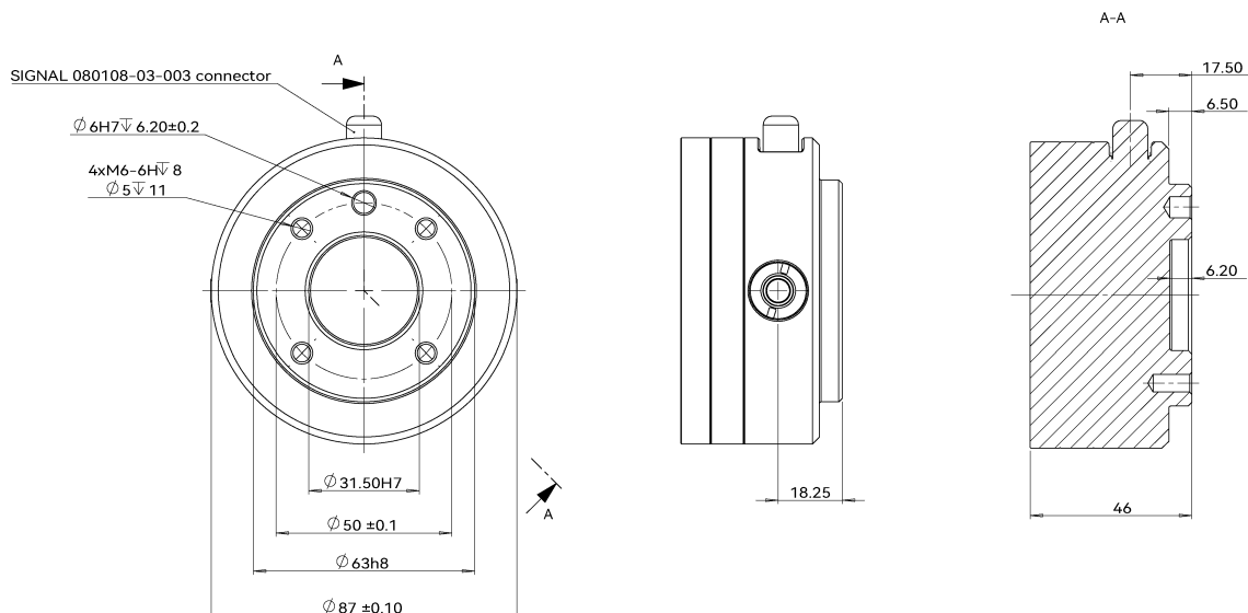
图 2-5: CS616 机器人工具法兰安装尺寸 (单位: mm)
