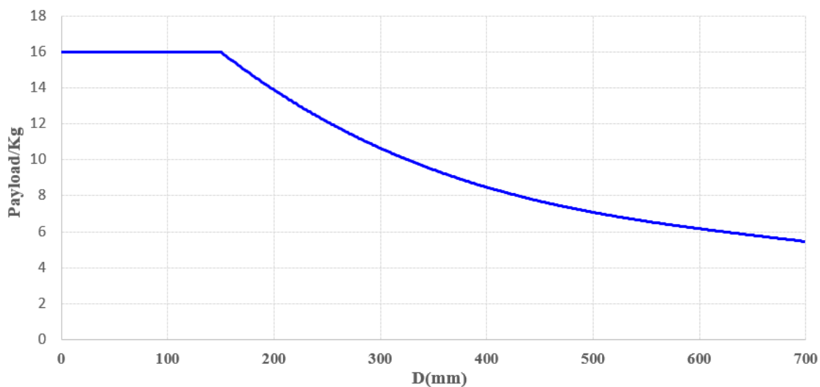
图 2-7: CS616 机器人有效负载
