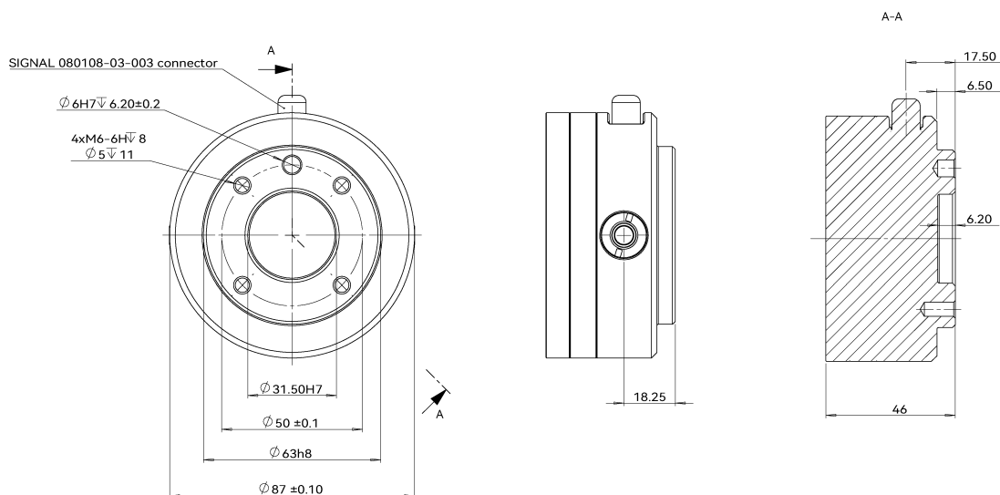
图 2-5: CS612 机器人工具法兰安装尺寸 (单位: mm)
