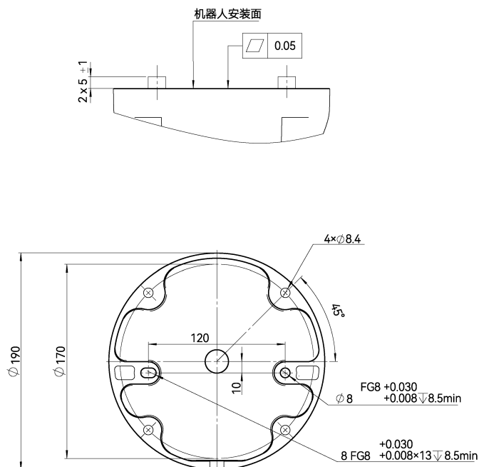
图 2-4: CS612 机器人基座安装尺寸 (单位: mm)
