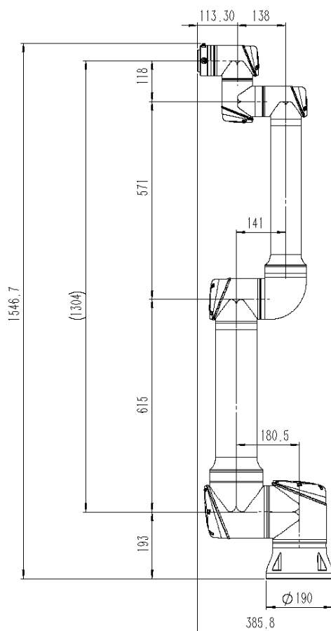
图 2-1: CS612 机器人机械尺寸（单位：mm）
