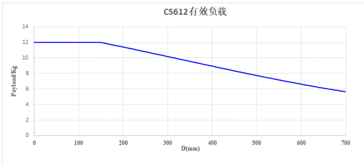
图 2-7: CS612 机器人有效负载
