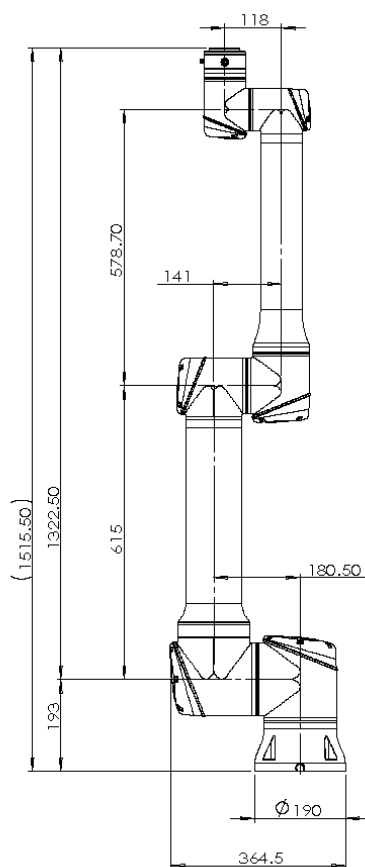
图 2-1: CS612A 机器人机械尺寸（单位：mm）
