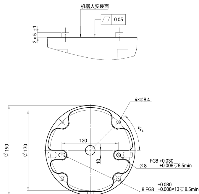
图 2-4: CS612A 机器人基座安装尺寸 (单位: mm)
