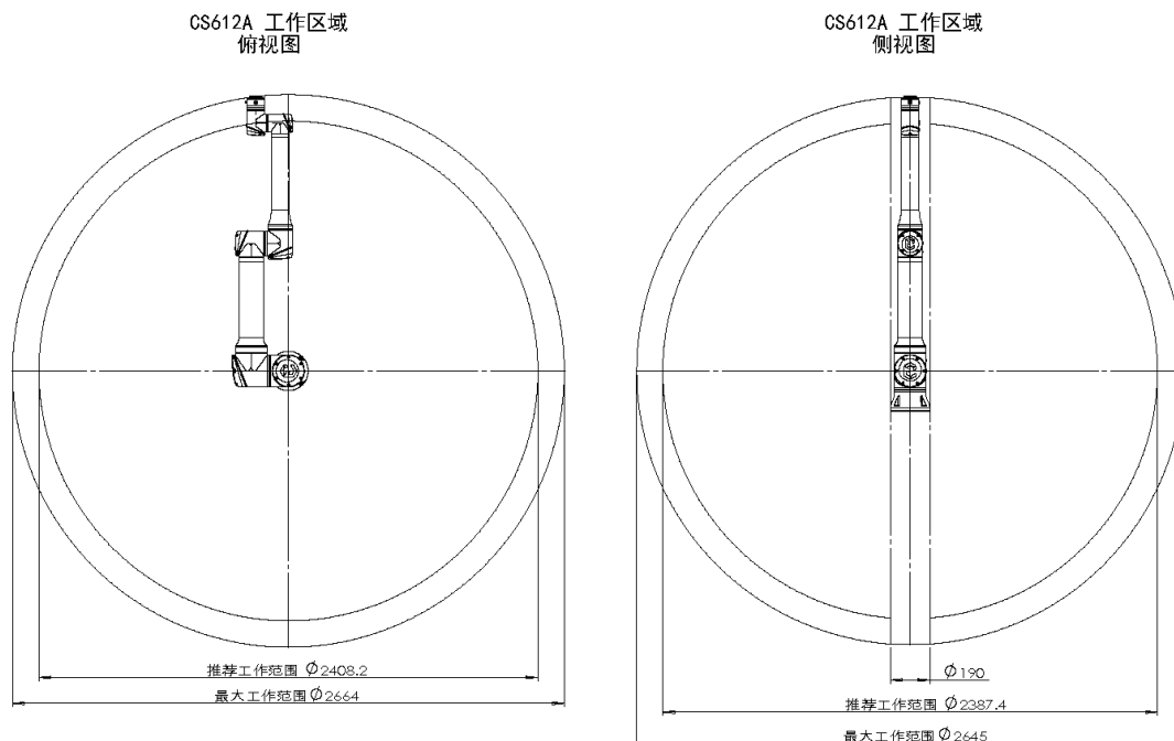
图 2-2: CS612A 机器人工作空间（单位：mm）
