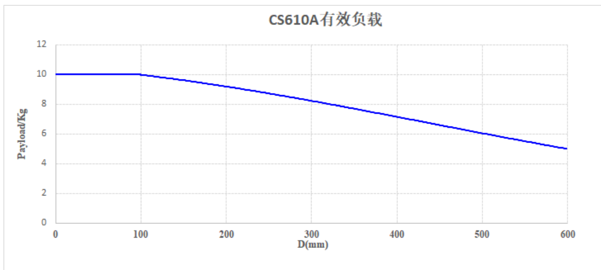
图 2-7: CS610A 机器人有效负载
