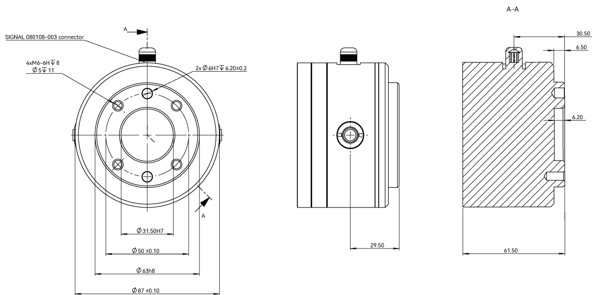
图 2-5: CS610A 机器人工具法兰安装尺寸 (单位: mm)
