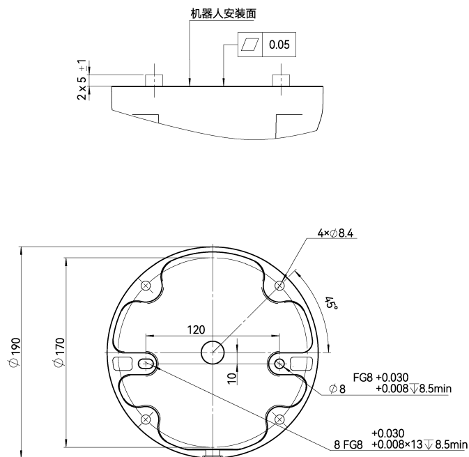
图 2-4: CS610A 机器人基座安装尺寸 (单位: mm)
