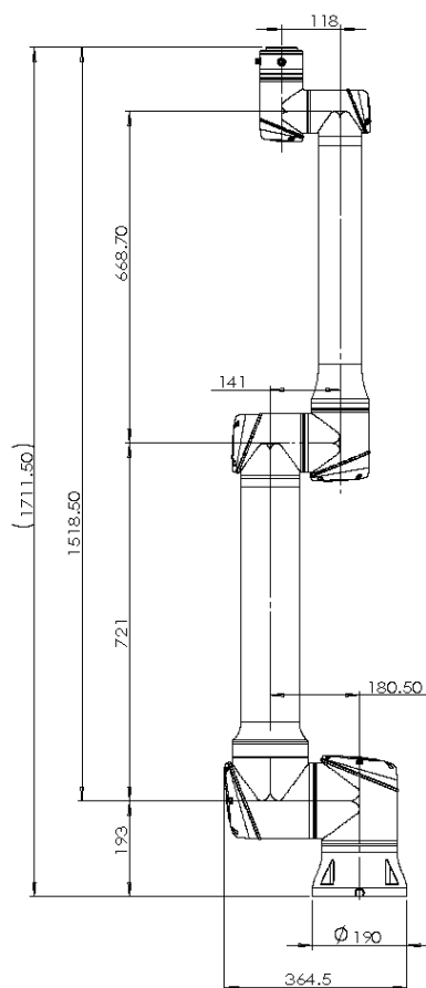
图 2-1: CS610A 机器人机械尺寸 (单位: mm)
