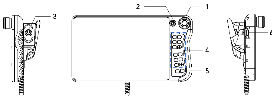
图 2-37: 示教器电气接口
