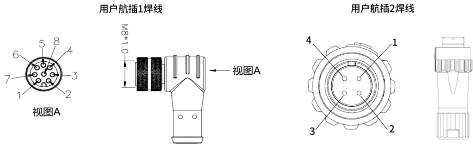
图 2-43: 用户航插焊线
