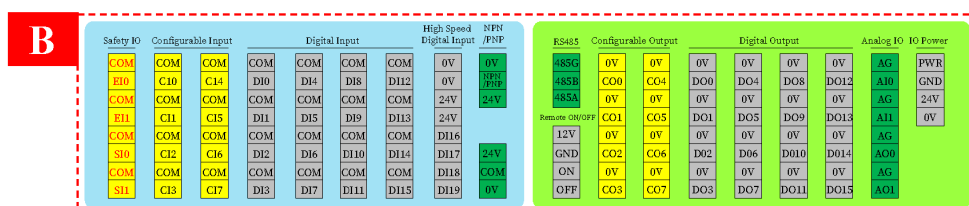
图 2-15: 控制柜内部电气接口 B 区
