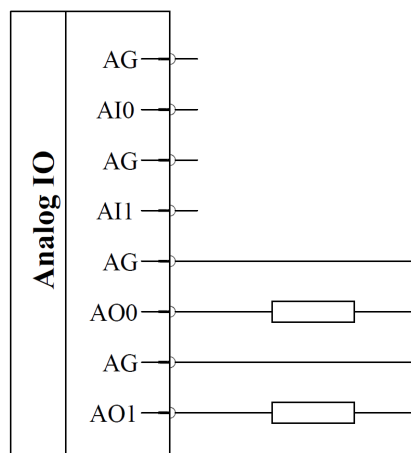
图 2-34: 模拟量输出连接方式
