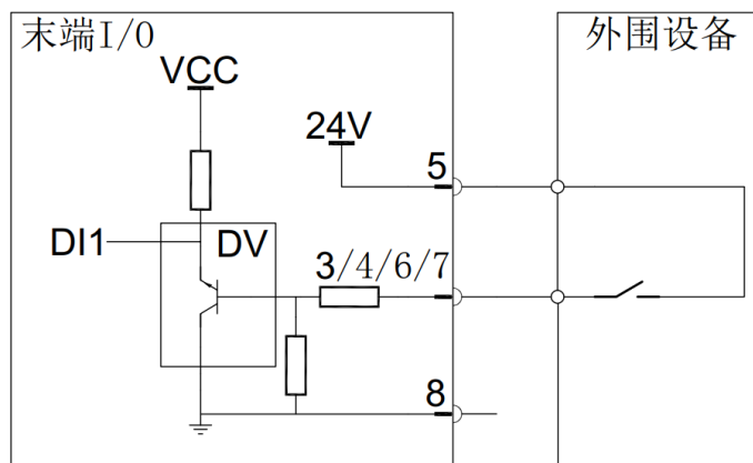
图 2-52: 工具数字输入接线方法
