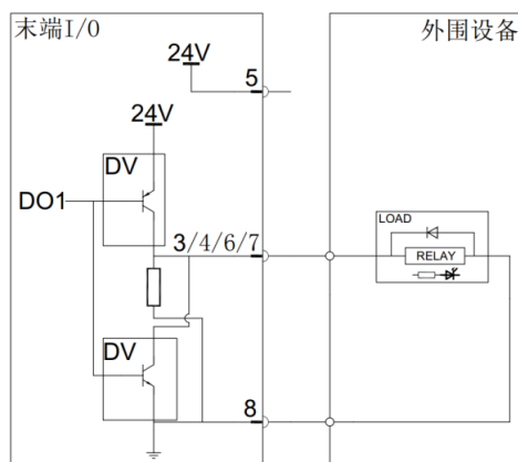
图 2-50: PNP 模式接线
