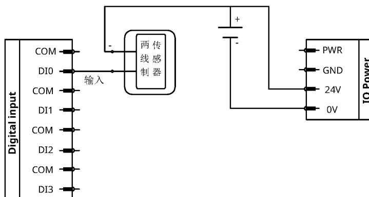
图 2-29: 数字输入 NPN 型接线 (外部供电)
