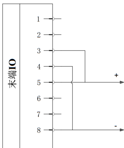
图 2-45: 双针模式 1 接线
