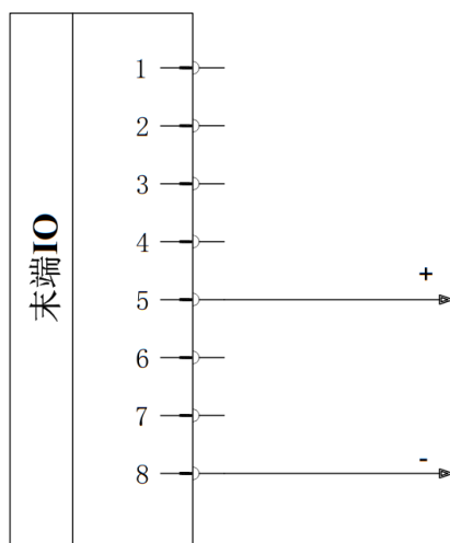
图 2-44: 单针电源模式接线
