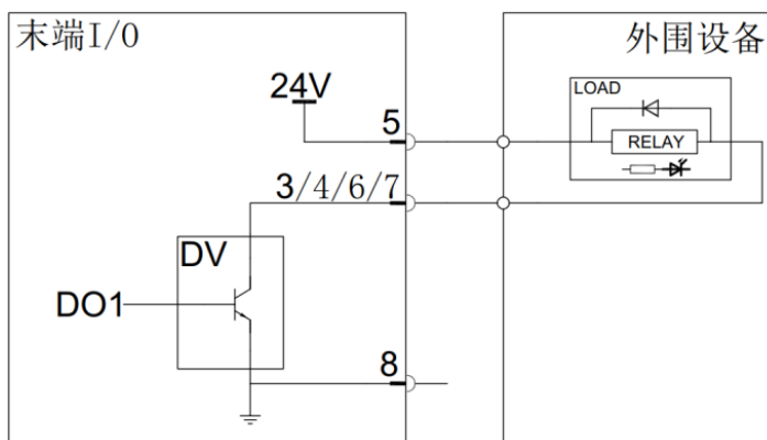
图 2-48: NPN 模式
