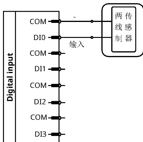
图 2-26: 数字输入 NPN 型接线 (内部供电)
