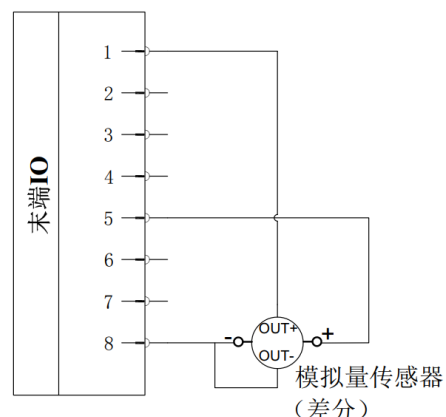
图 2-54: 模拟输入（差分）连接
