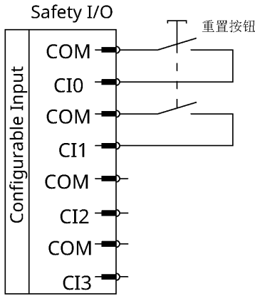
图 2-23: 控制柜的重置按钮连接方式
