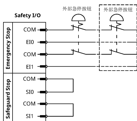
图 2-21: 单个或多个外部急停按钮连接
