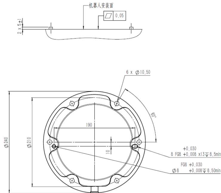
图 2-4: CS530H 机器人基座安装尺寸 (单位: mm)
