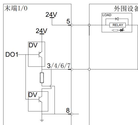
图 2-51: NPN 模式接线
