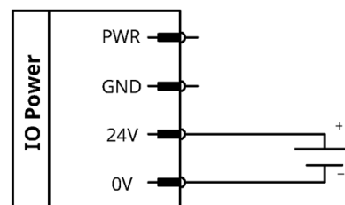
图 2-36: 使用外部电源接线方式
