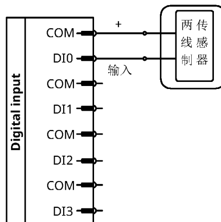
图 2-27: 数字输入 PNP 型接线 (内部供电)
