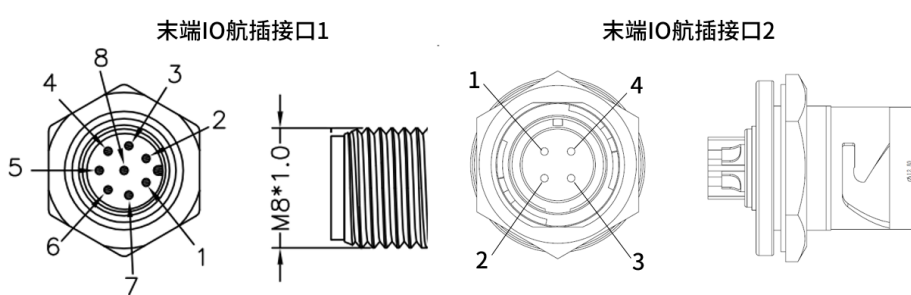
图 2-42: 机器人末端 I/O 航空插接口
