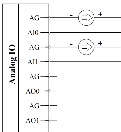
图 2-33: 模拟量输入连接方式
