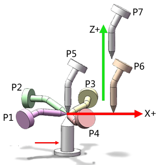
图 3-50: 三点法示教坐标系方向
