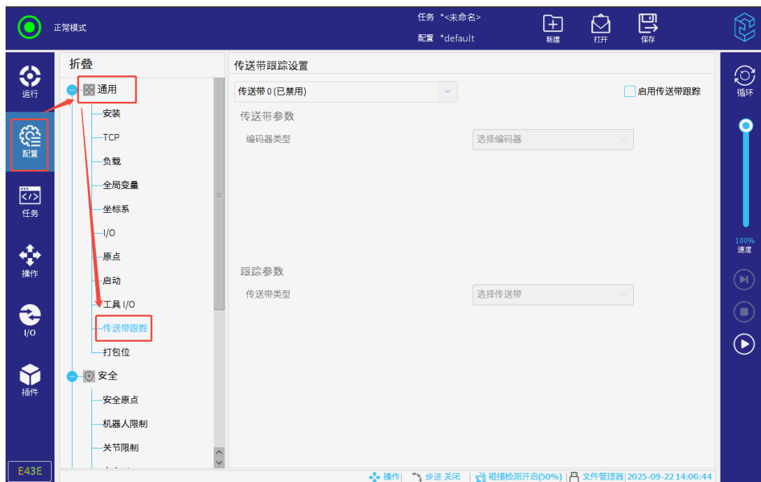
图 3-73: 传送带跟踪：绝对式
