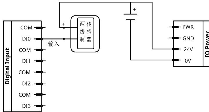
图 2-30: 数字输入 PNP 型接线（外部供电）
