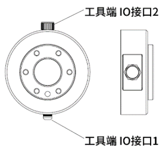
图 2-41: 机器人末端 I/O
