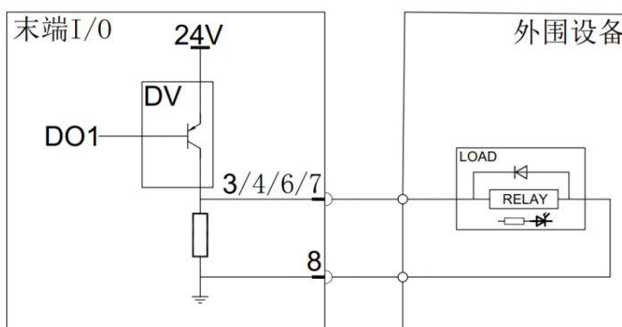
图 2-49: PNP 模式
