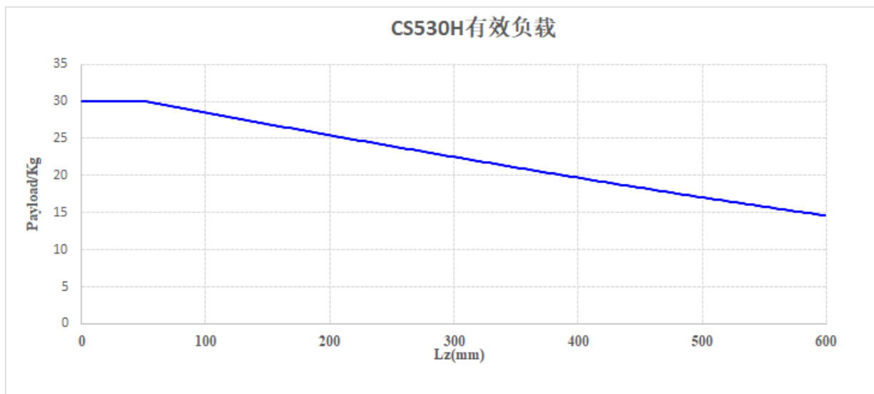
图 2-7: CS530H 机器人有效负载
