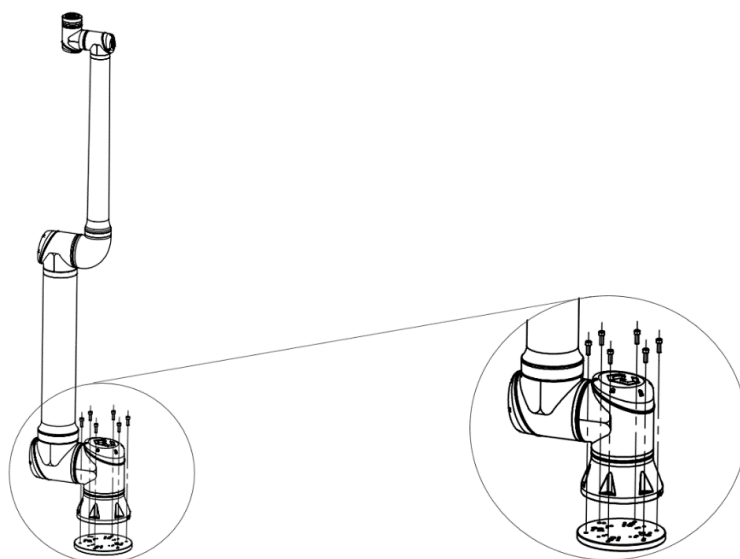
图 1-3: 本体安装
