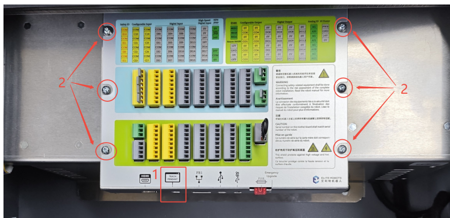
图 2-8: 拆除或断开位置
