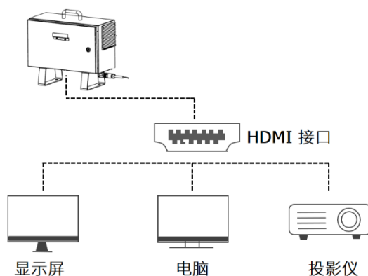
图 2-14: HDMI 接口
