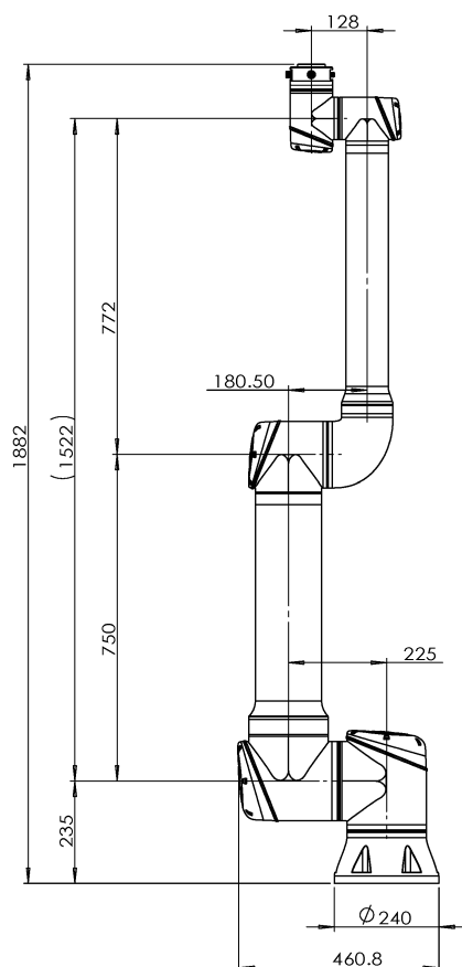
图 2-1: CS530H 机器人机械尺寸 (单位: mm)
