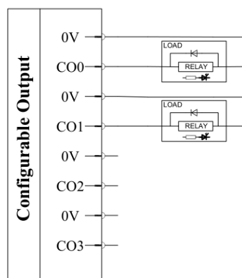
图 2-25: 配置输出接线方式
