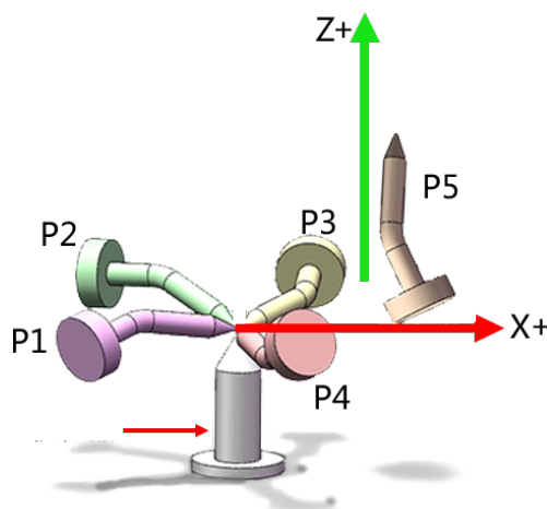
图 3-48: 工具坐标设定
