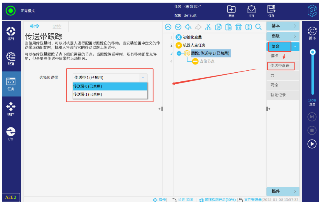
图 3-156: 传送带
