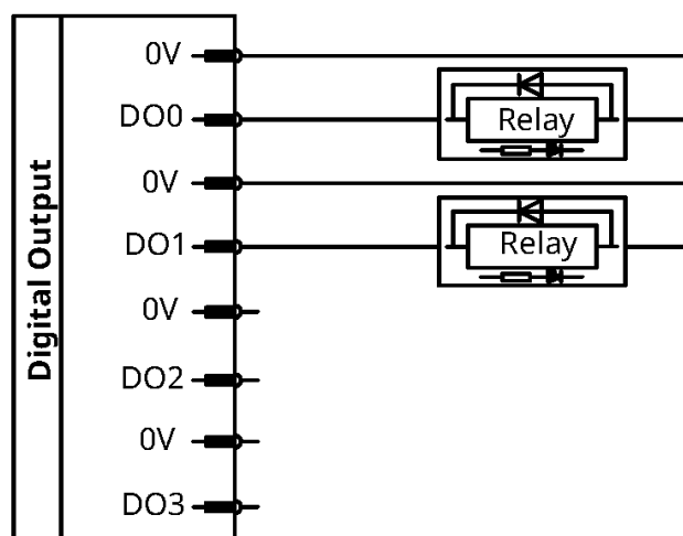
图 2-28: 数字输出接线方式 (内部供电)
