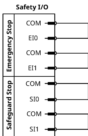
图 2-20: 安全 I/O 默认配置连接
