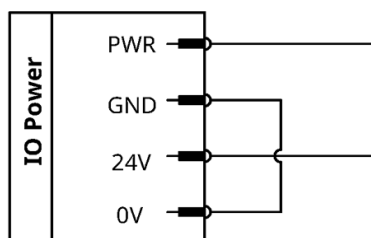
图 2-35: 使用内部电源接线方式
