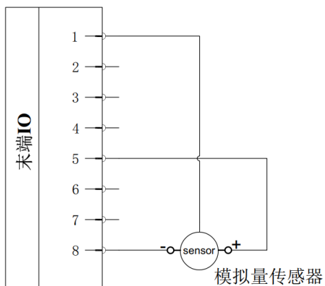
图 2-53: 模拟输入（非差分）连接
