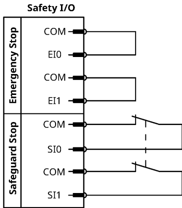
图 2-22: 控制柜的防护停止装置连接
