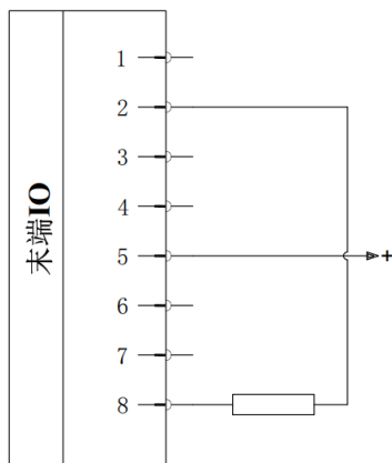
图 2-55: 模拟输出（非差分）连接
