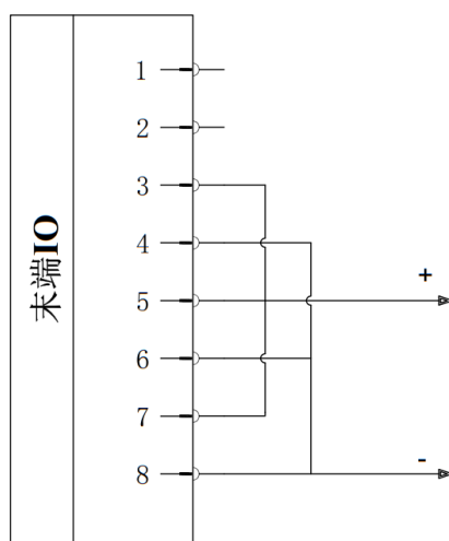
图 2-47: 三针电源模式
