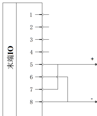
图 2-46: 双针模式 2 接线
