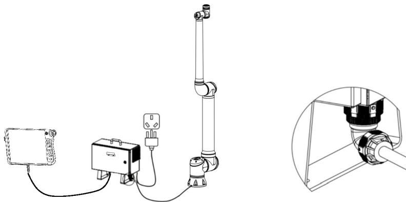
图 1-6: 整机安装-本体电缆锁定
