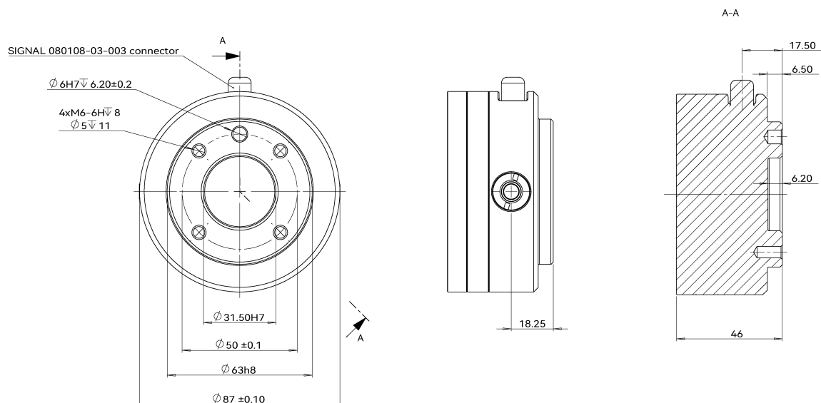
图 2-5: CS520H 机器人工具法兰安装尺寸 (单位: mm)
