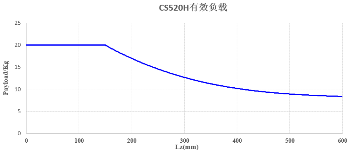
图 2-7: CS520H 机器人有效负载
