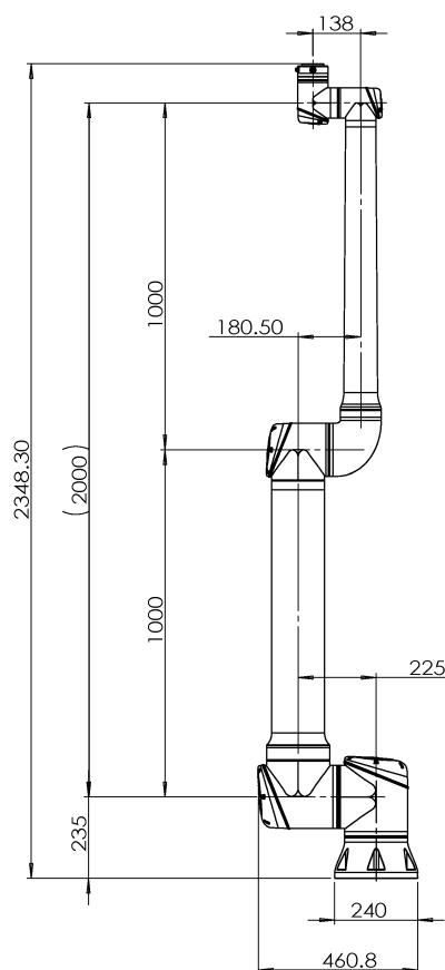
图 2-1: CS520H 机器人机械尺寸（单位：mm）
