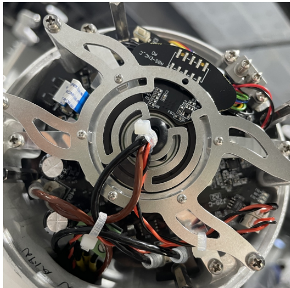
图 3-14: 重连电线
