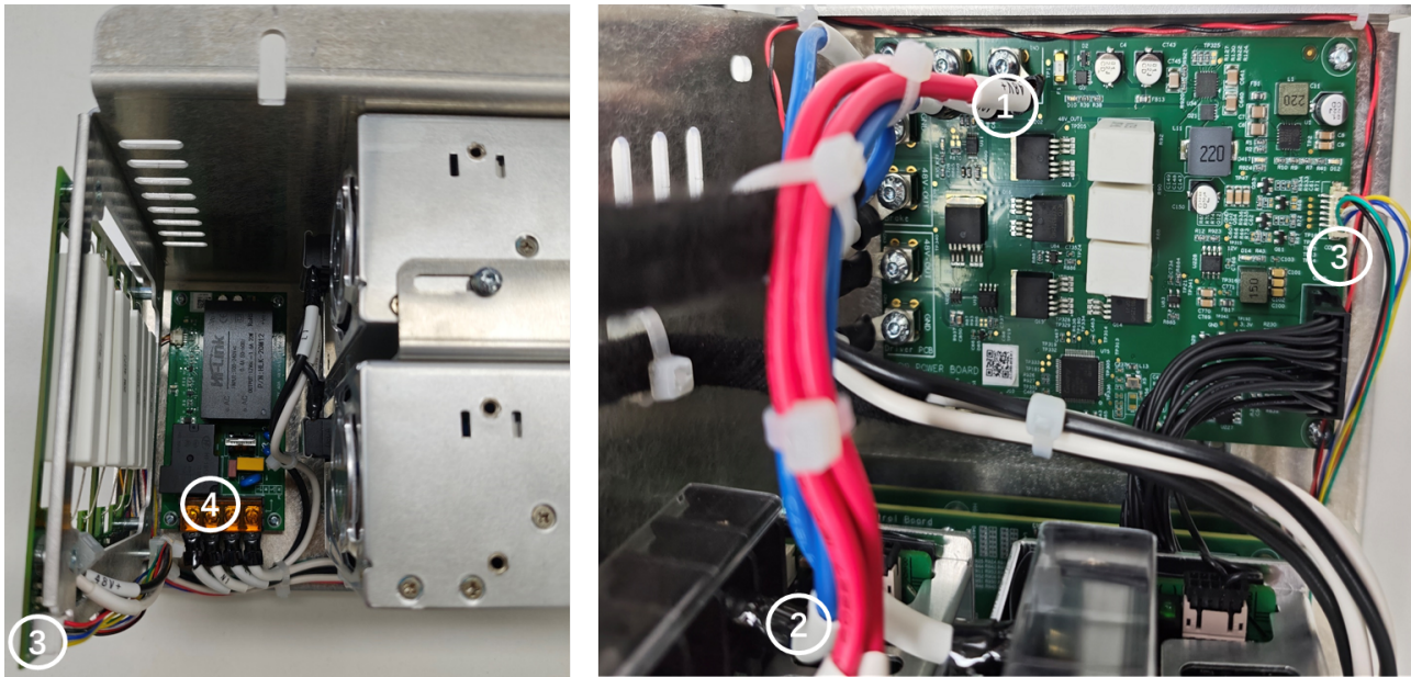
图 3-26: 控制柜上的电源连接线位置
