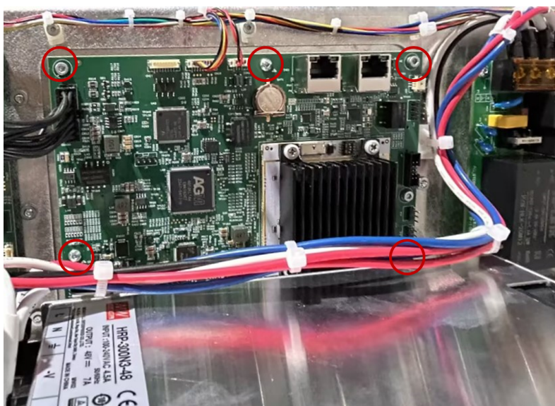
图 3-28: 螺钉位置
