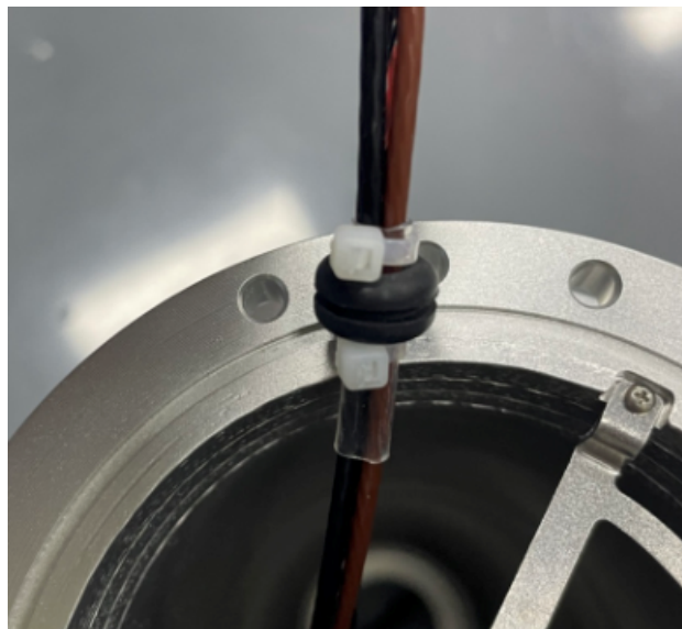
图 3-21: 扎线
