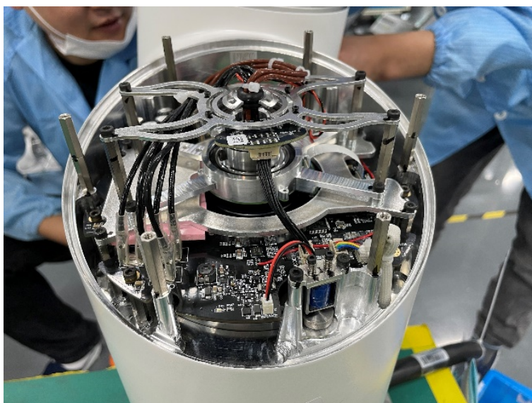
图 3-9: 重连电线
