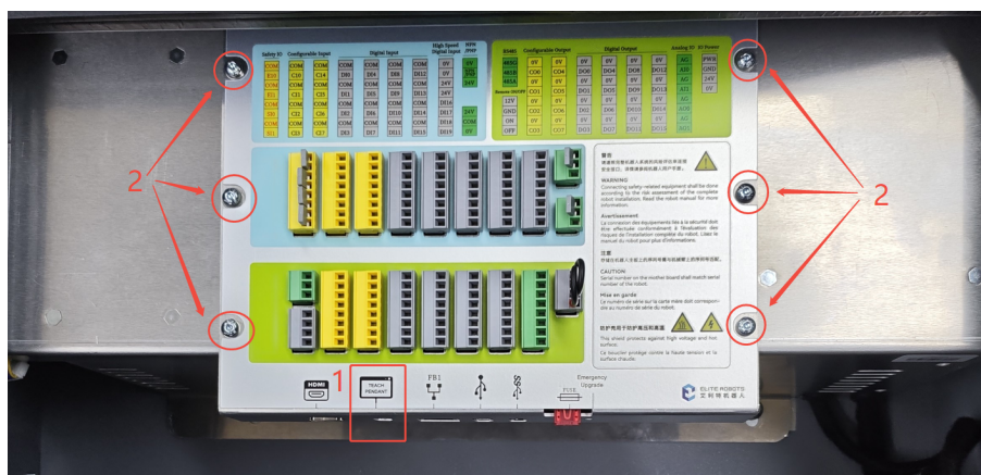
图 3-33: 拆除或断开位置
