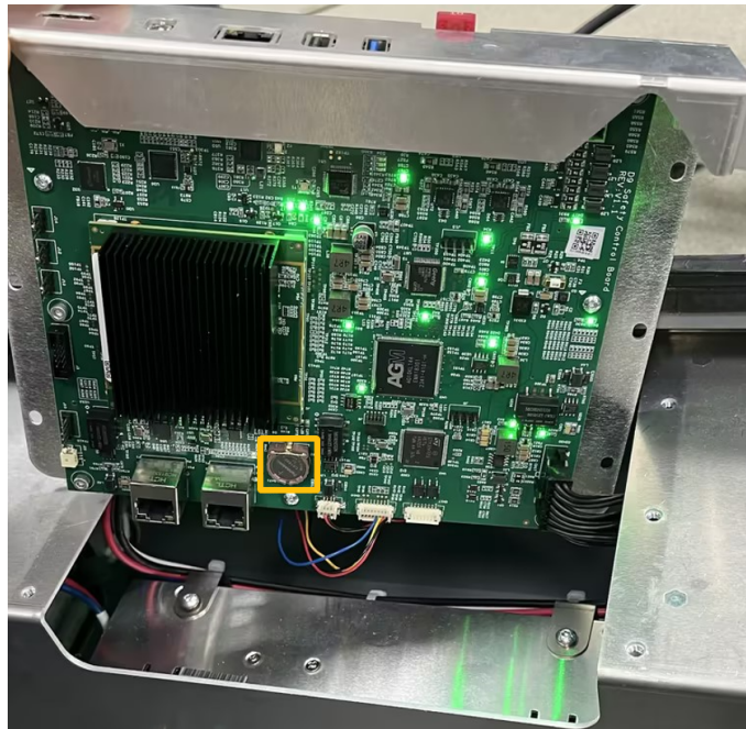
图 3-34: 纽扣电池安装位置
