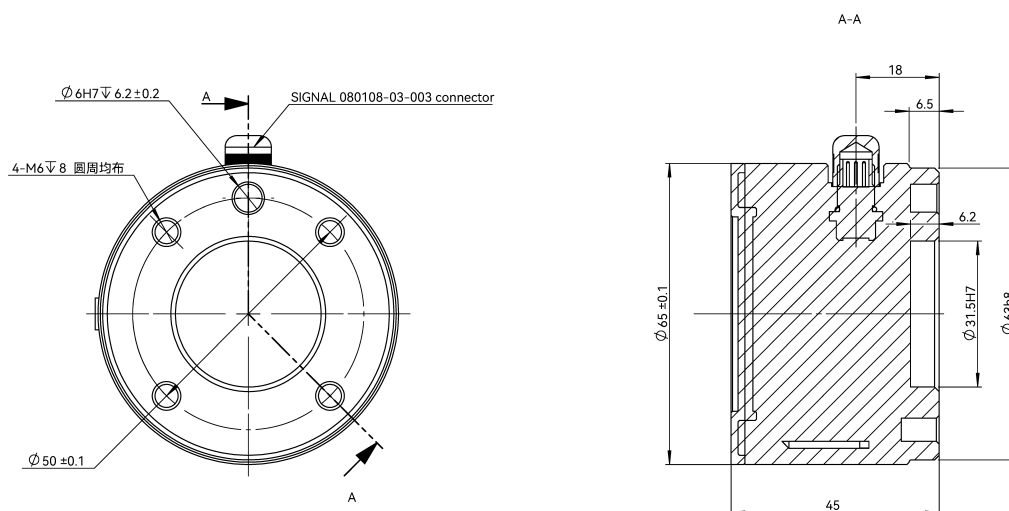
图 2-5: LS65 机器人工具法兰安装尺寸图，单位 mm
