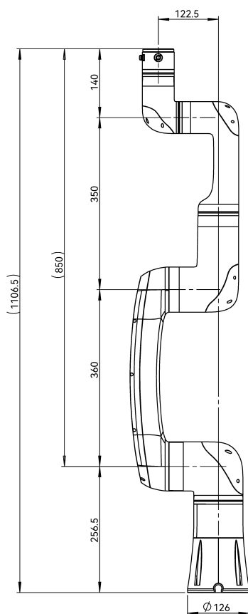
图 2-1: LS65 机器人机械尺寸图，单位 mm
