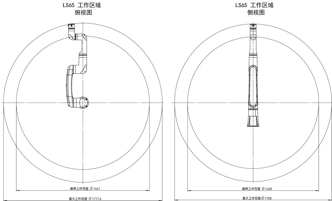
图 2-2: LS65 机器人工作空间，单位 mm
