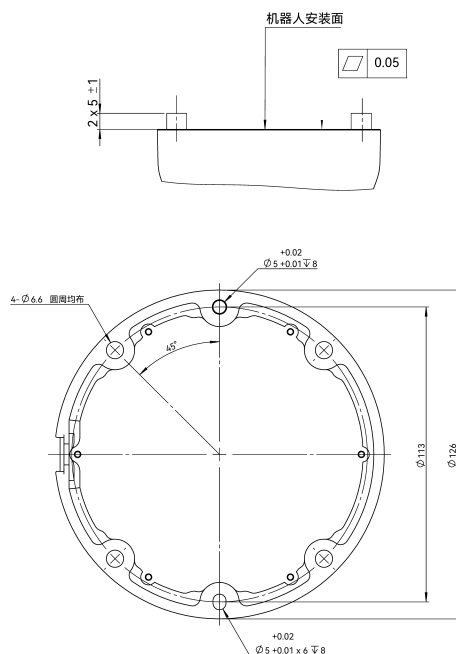
图 2-4: LS65 机器人基座安装尺寸图，单位 mm
