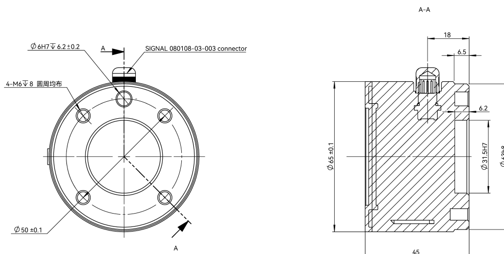
图 2-5: LS62 机器人工具法兰安装尺寸图，单位 mm
