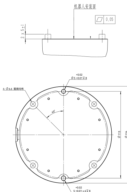
图 2-4: LS62 机器人基座安装尺寸图，单位 mm
