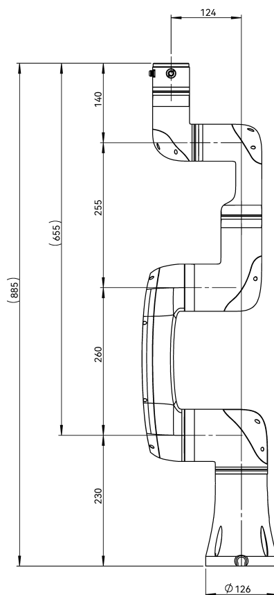
图 2-1: LS62 机器人机械尺寸图，单位 mm
