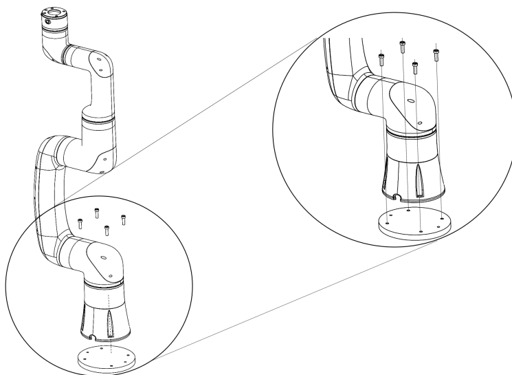
图 1-3: 本体安装
