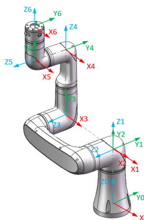
图 2-3: 机器人 DH 示意图
