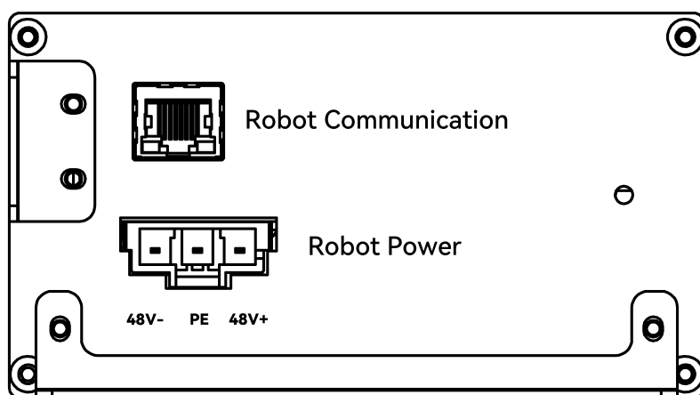
图 2-9: 本体通讯、供电接口示意图
