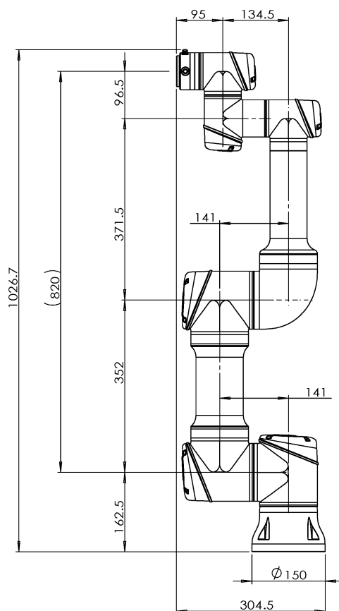
图 2-1: CS68 机器人机械尺寸图，单位 mm
