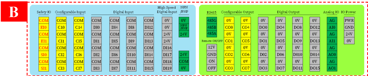
图 2-15: 控制柜内部电气接口 B 区
