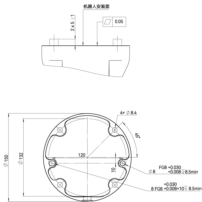
图 2-4: CS68 机器人基座安装尺寸图，单位 mm
