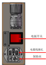
图 2-10: 电源输入插座
