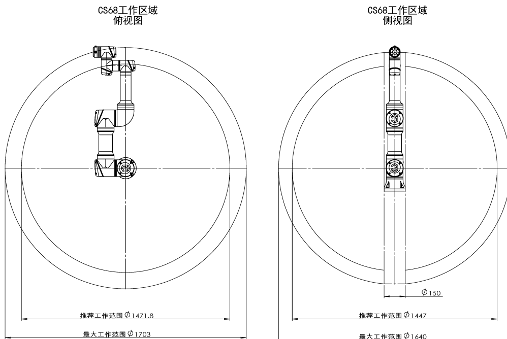
图 2-2: CS68 机器人工作空间，单位 mm
