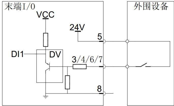
图 2-52: 工具数字输入接线方法
