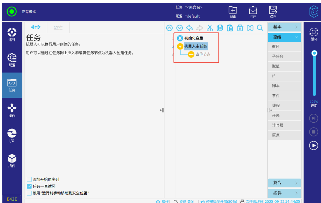
图 3-102: 任务树
