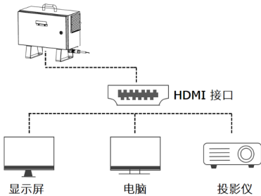
图 2-14: HDMI 接口
