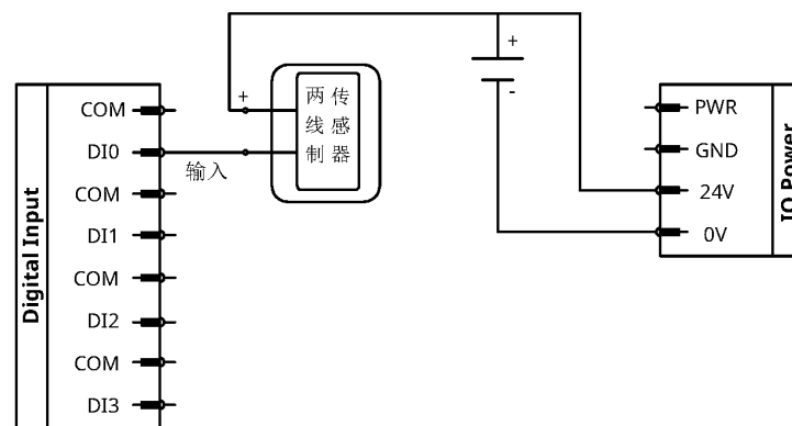
图 2-30: 数字输入 PNP 型接线（外部供电）
