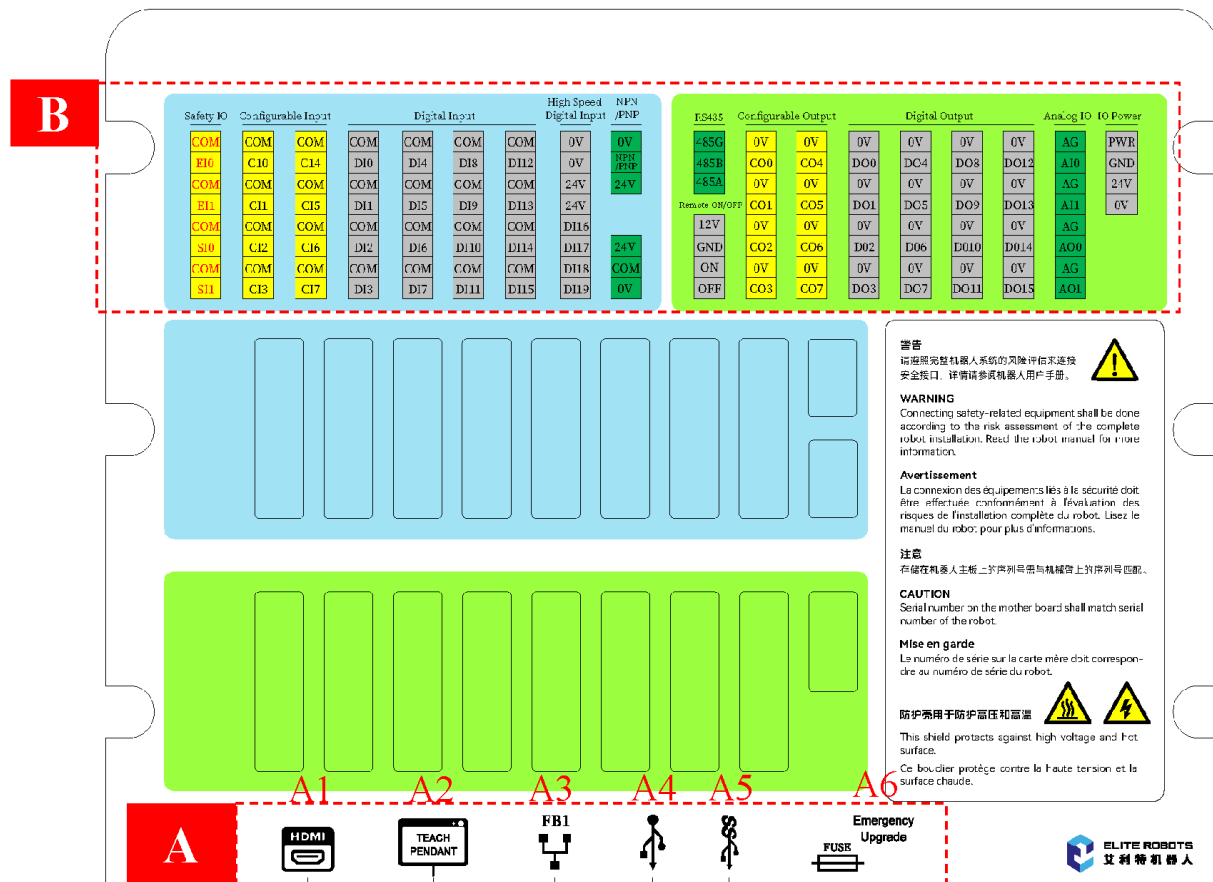
图 2-13: 控制柜内部电气接口示意图
