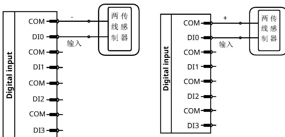
图 2-26: 数字输入 NPN 型接线 (内部供电) 图 2-27: 数字输入 PNP 型接线 (内部供电)
