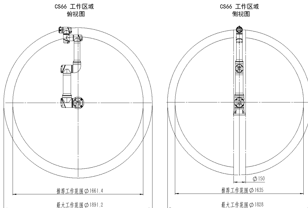
图 2-2: CS66 机器人工作空间，单位 mm
