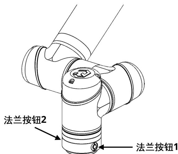
图 2-6: CS66 机器人末端法兰按钮
