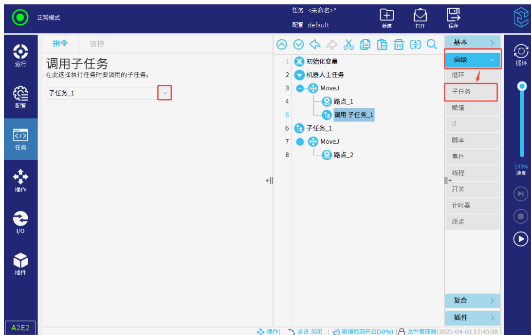
图 3-124: 调用子任务
