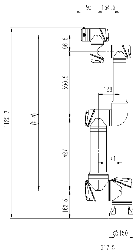
图 2-1: CS66 机器人机械尺寸图，单位 mm
