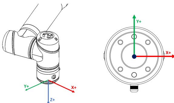
图 3-42: 工具坐标默认方向
