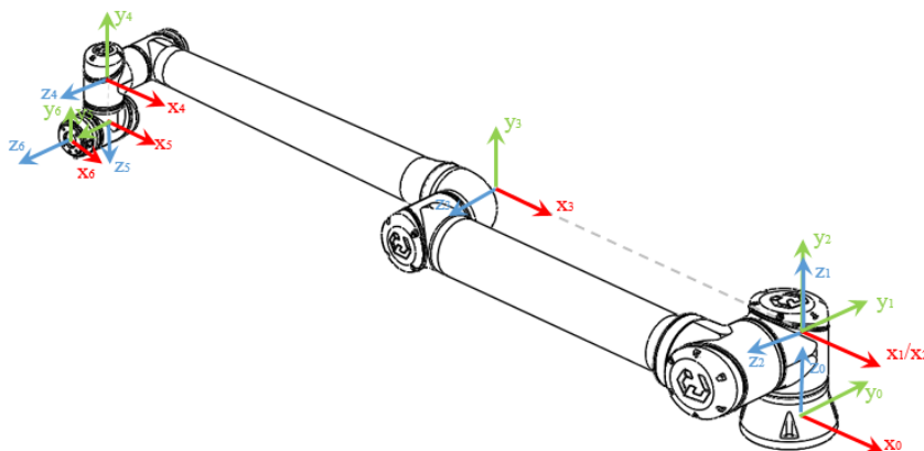
图 2-3: 机器人 DH 示意图
