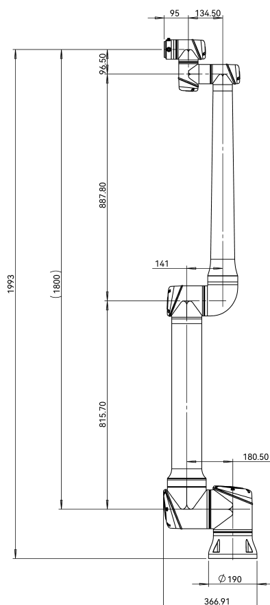
图 2-1: CS66-18 机器人机械尺寸图，单位 mm
