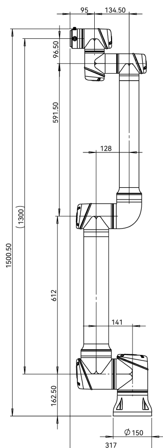
图 2-1: CS64-13 机器人机械尺寸图，单位 mm
