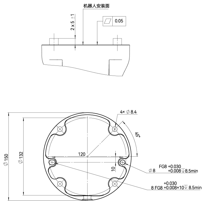
图 2-4: CS64-13 机器人基座安装尺寸图，单位 mm
