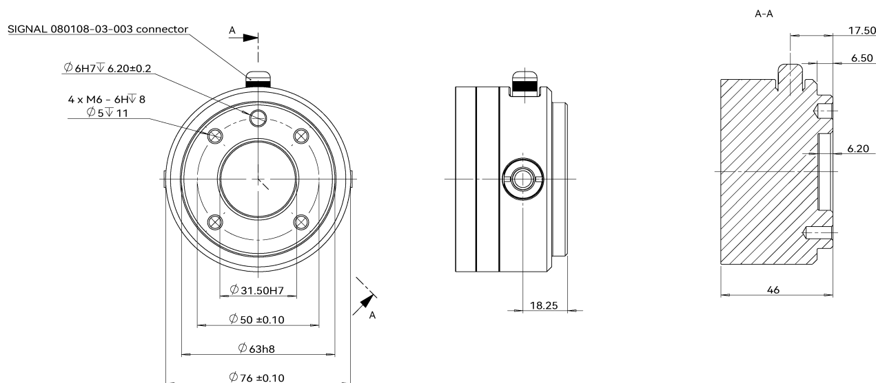
图 2-5: CS64-13 机器人工具法兰安装尺寸图，单位 mm
