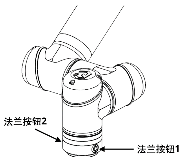
图 2-6: CS64-13 机器人末端法兰按钮
