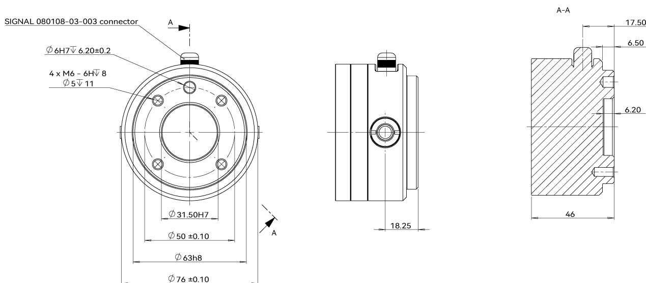
图 2-5: CS63 机器人工具法兰安装尺寸图，单位 mm
