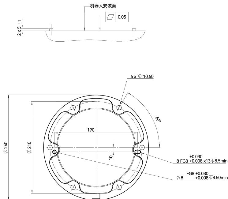
图 2-4: CS630 机器人基座安装尺寸图, 单位 mm
