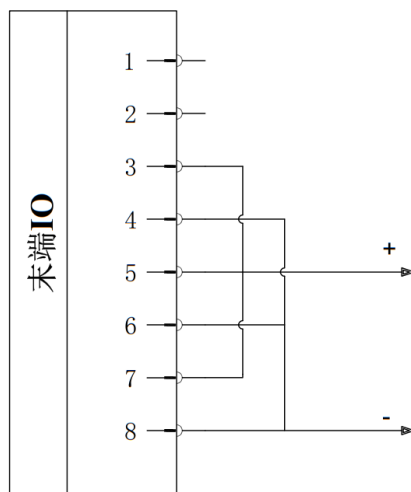
图 2-47: 三针电源模式
