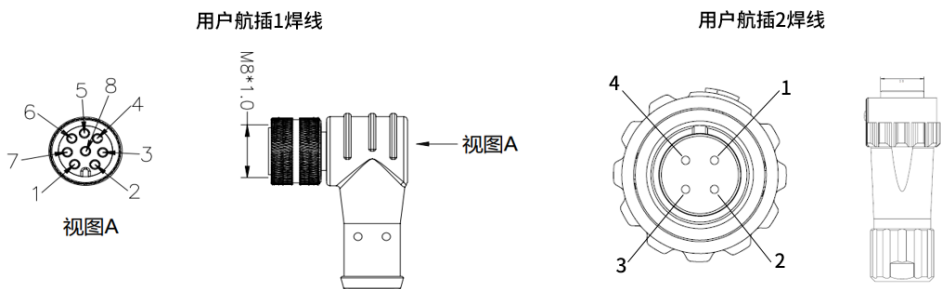
图 2-43: 用户航空插头焊线
