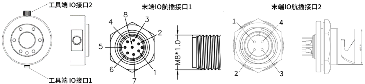
图 2-41: 机器人末端 I/O
