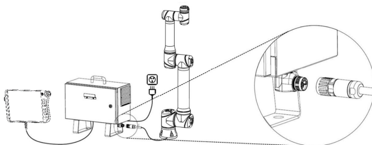
图 1-5: 整机安装-本体电缆未连接
