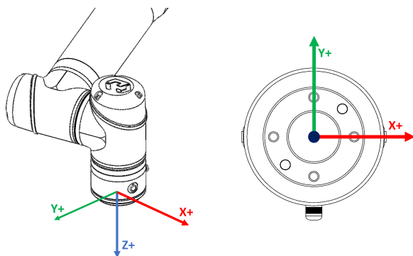
图 3-42: 工具坐标默认方向
