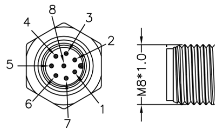
图 2-42: 机器人末端 I/O 航空插接口
