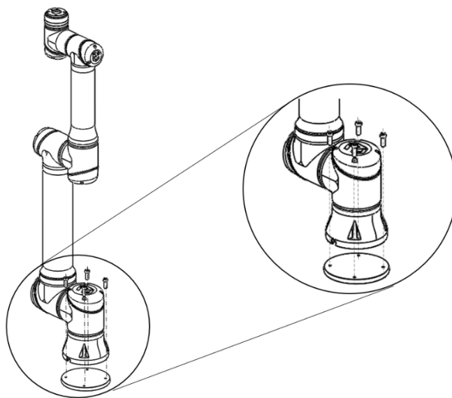
图 1-3: 本体安装
