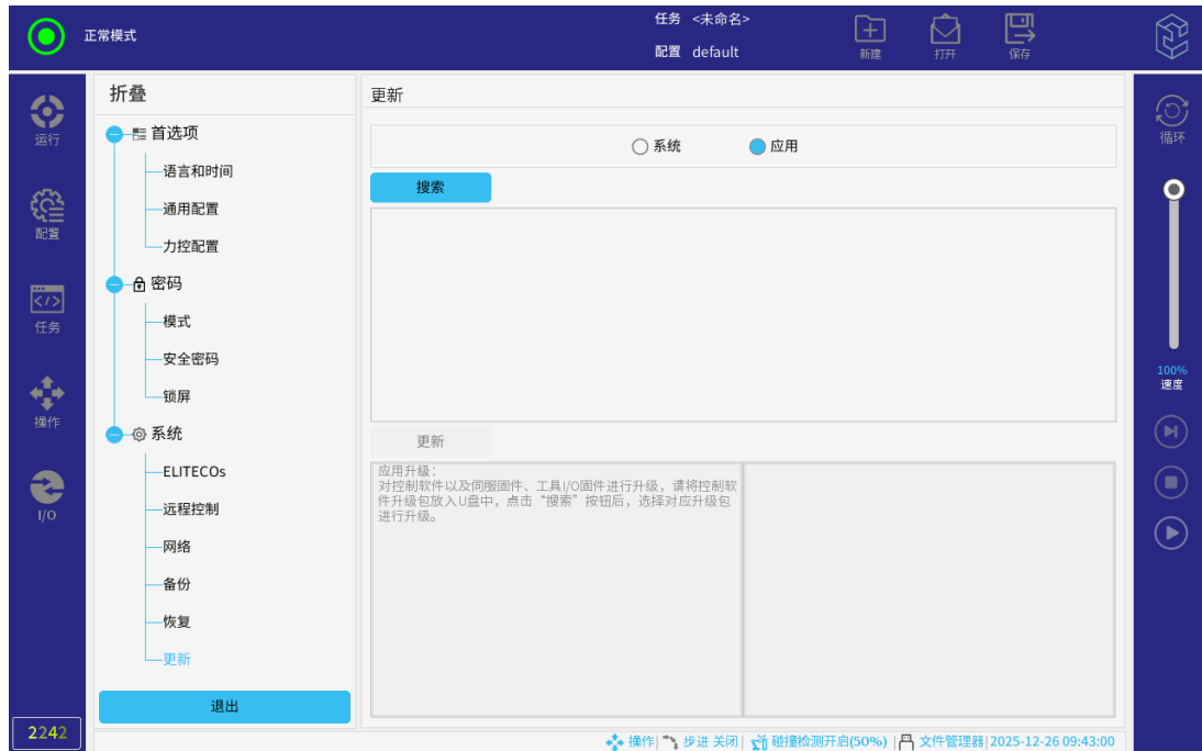
图 3-34: 更新
