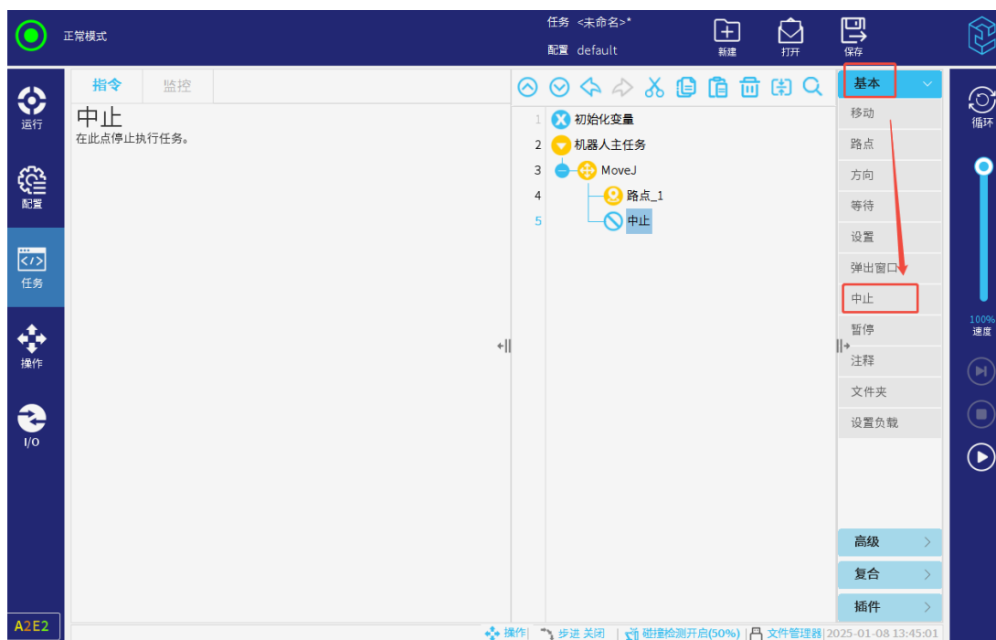
图 3-118: 中止
