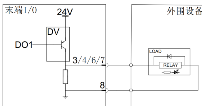
图 2-49: PNP 模式
