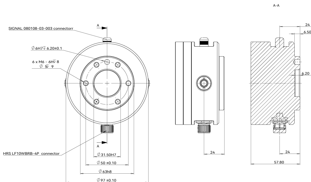
图 2-5: CS530H 机器人工具法兰安装尺寸图, 单位 mm
