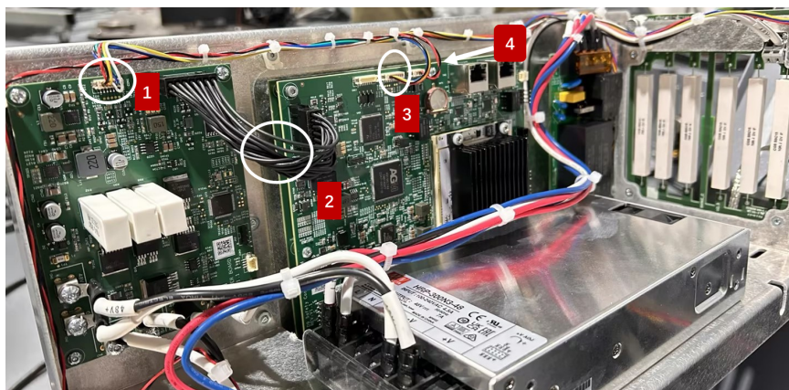
图 3-28: 电源板、刹车板到 Safe IO 的线缆位置
