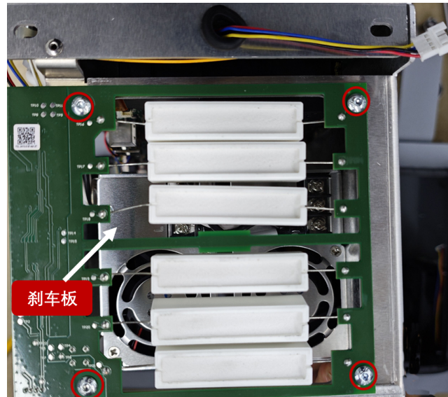
图 3-32: 取下刹车板
