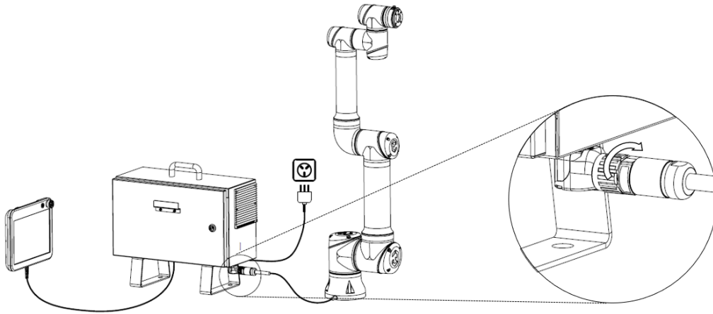
图 1-6: 整机安装-本体电缆连接
