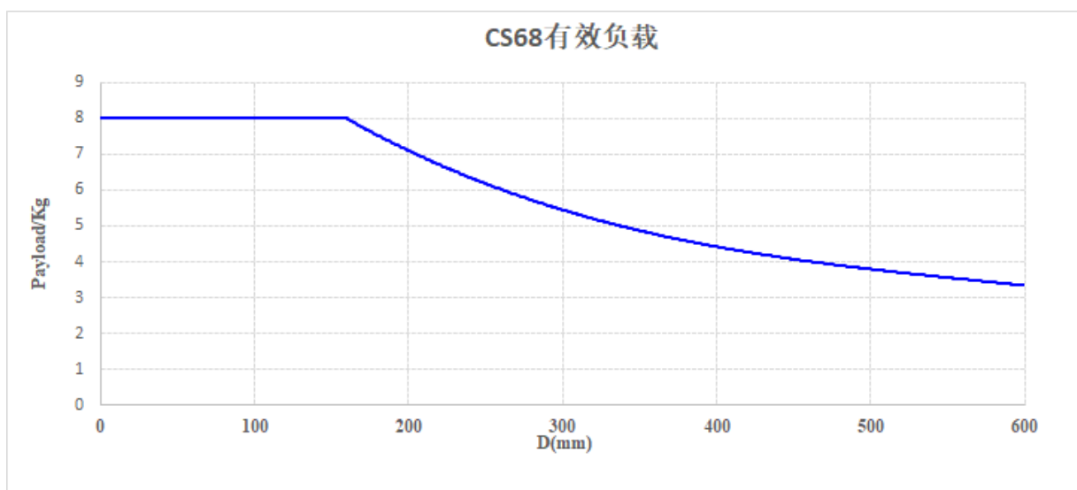
图 2-7: 有效负载图
