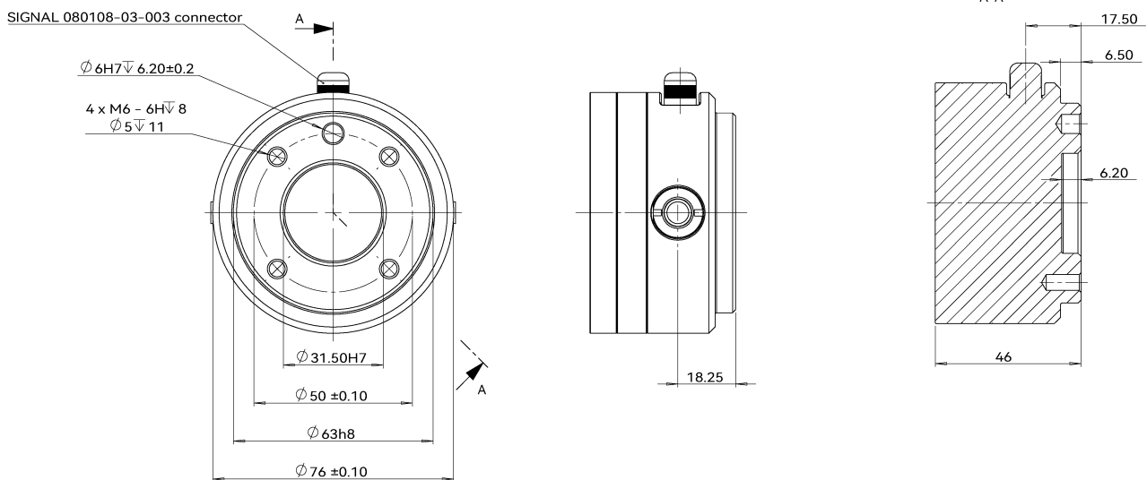
图 2-5: CS68 机器人工具法兰安装尺寸图, 单位 mm
