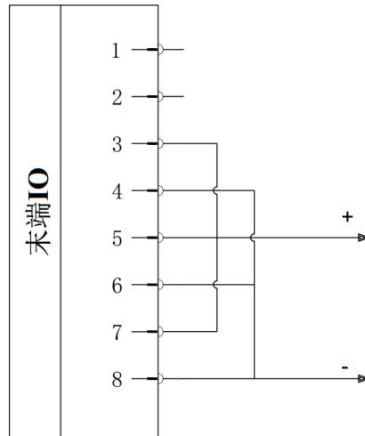
图 2-45: 三针电源模式
