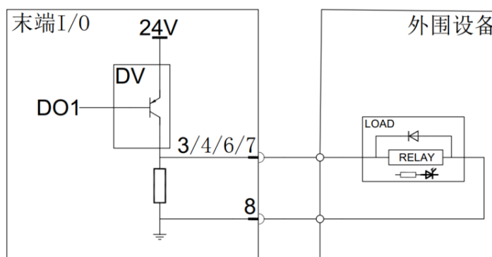
图 2-47: PNP 模式
