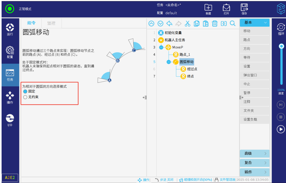
图 3-107: 圆弧运动
