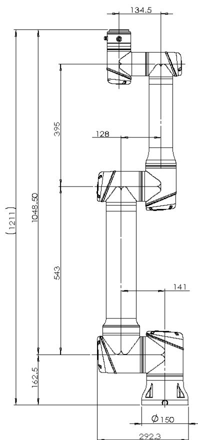
图 2-1: CS66AZ 机器人机械尺寸图，单位 mm
