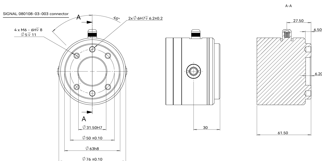
图 2-5: CS66AZ 机器人工具法兰安装尺寸图，单位 mm
