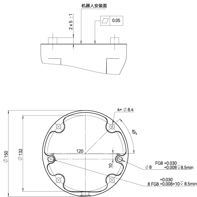
图 2-4: CS66A 机器人基座安装尺寸图，单位 mm
