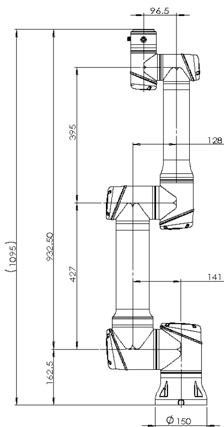
图 2-1: CS66A 机器人机械尺寸图，单位 mm
