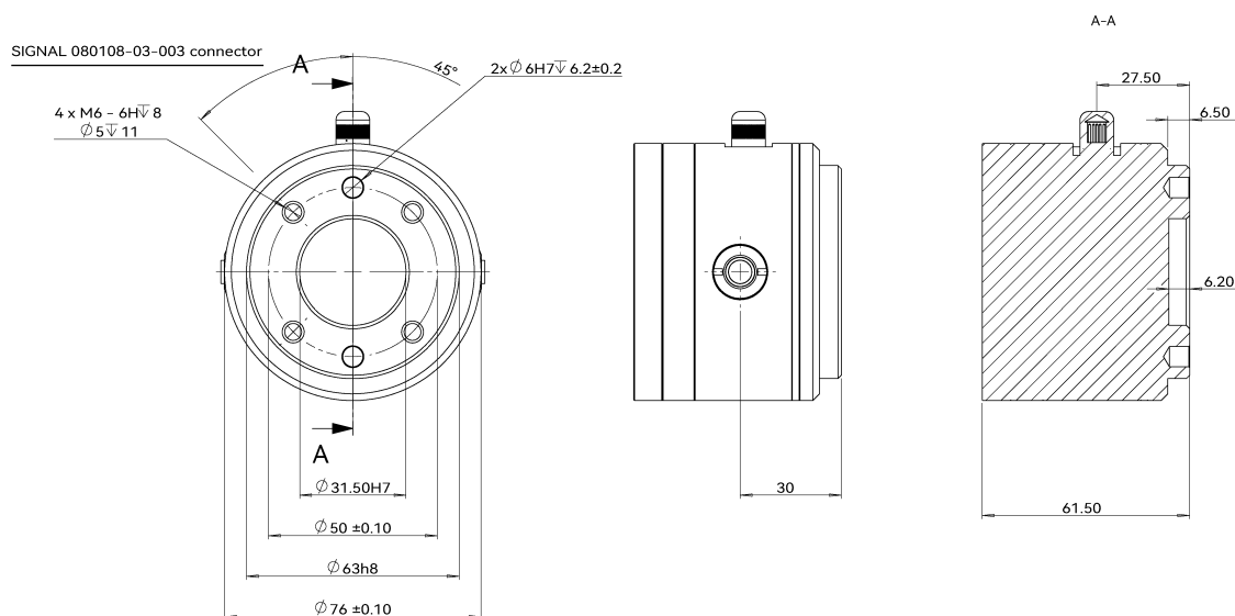
图 2-5: CS66A 机器人工具法兰安装尺寸图，单位 mm
