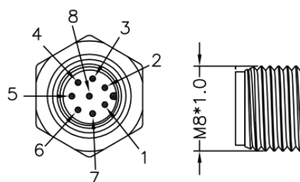
图 2-40: 机器人末端 I/O 航空插接口
