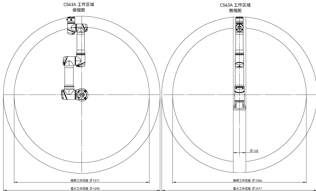
图 2-2: CS63A 机器人工作空间，单位 mm
