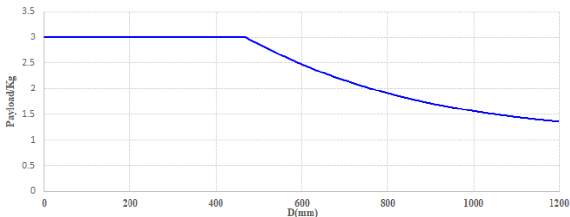
图 2-7: 有效负载图
