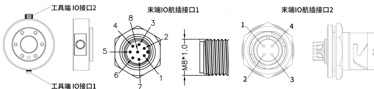
图 2-32: 机器人末端 I/O 航空插接口
