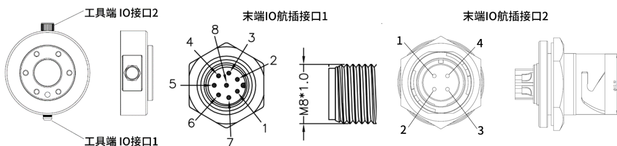
图 2-31: 机器人末端 I/O
