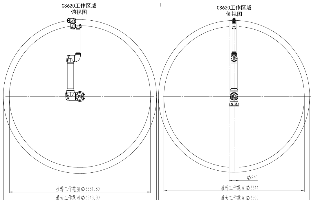
图 2-2: CS620 机器人工作空间，单位 mm
