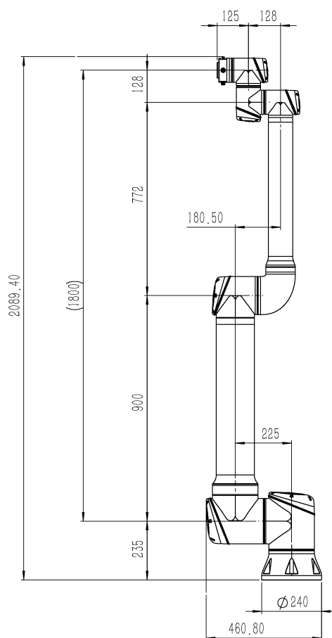
图 2-1: CS620 机器人机械尺寸图，单位 mm
