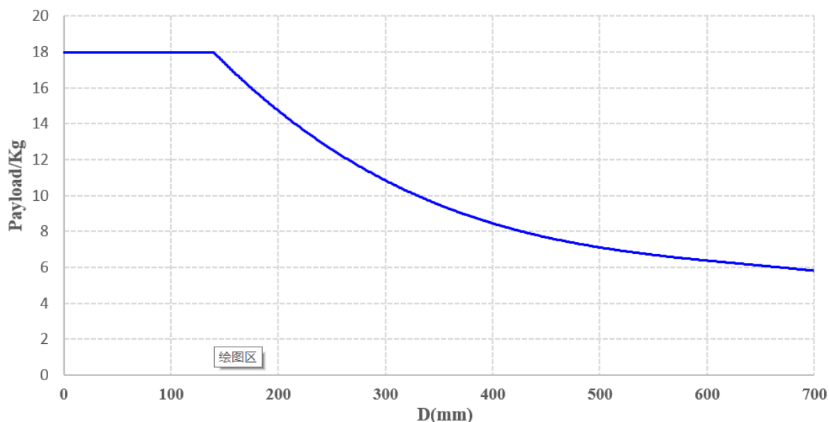
图 2-7: 有效负载图
