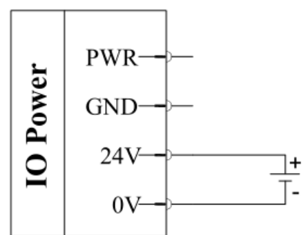
图 2-20: 使用外部电源接线方式
