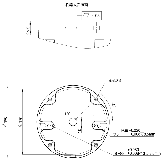
图 2-4: CS618 机器人基座安装尺寸图，单位 mm
