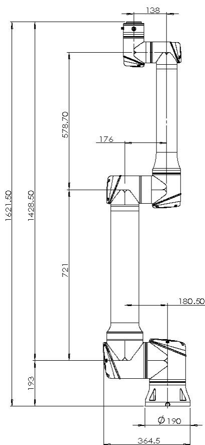
图 2-1: CS612AZ 机器人机械尺寸图，单位 mm
