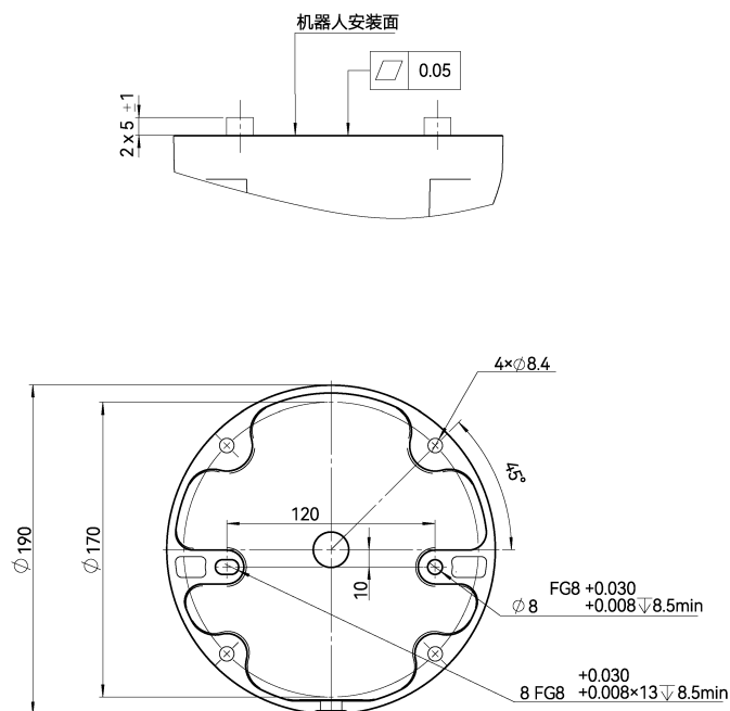
图 2-4: CS612AZ 机器人基座安装尺寸图, 单位 mm
